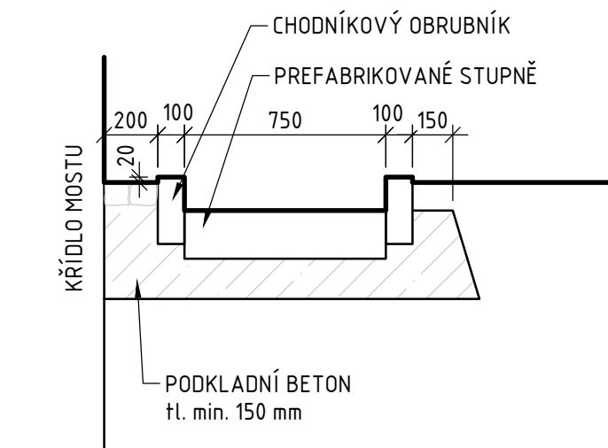
ŘEZ A-A 1:25
