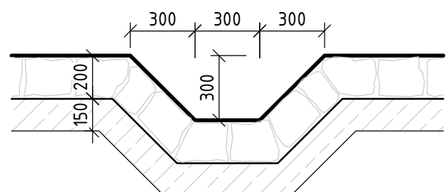
PŘÍČNÝ ŘEZ SKLUZEM Z LOMOVÉHO KAMENE 1:25
