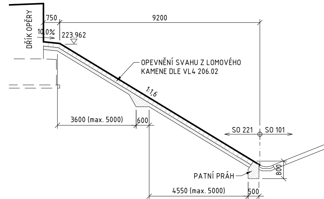
PODÉLNÝ ŘEZ ODLÁŽDĚNÍM POD MOSTEM 1:100
