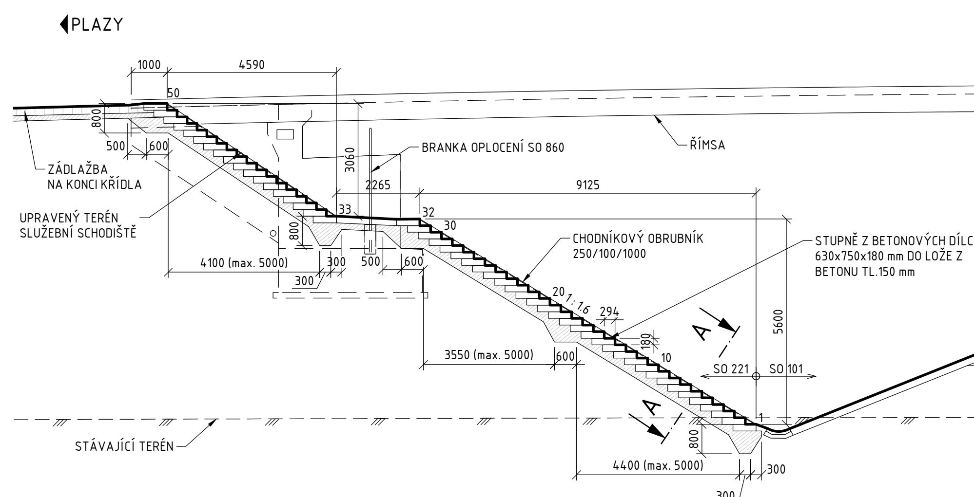
SLUŽEBNÍ SCHODIŠTĚ PODÉL KŘÍDLA OPĚRY 01 1:100
