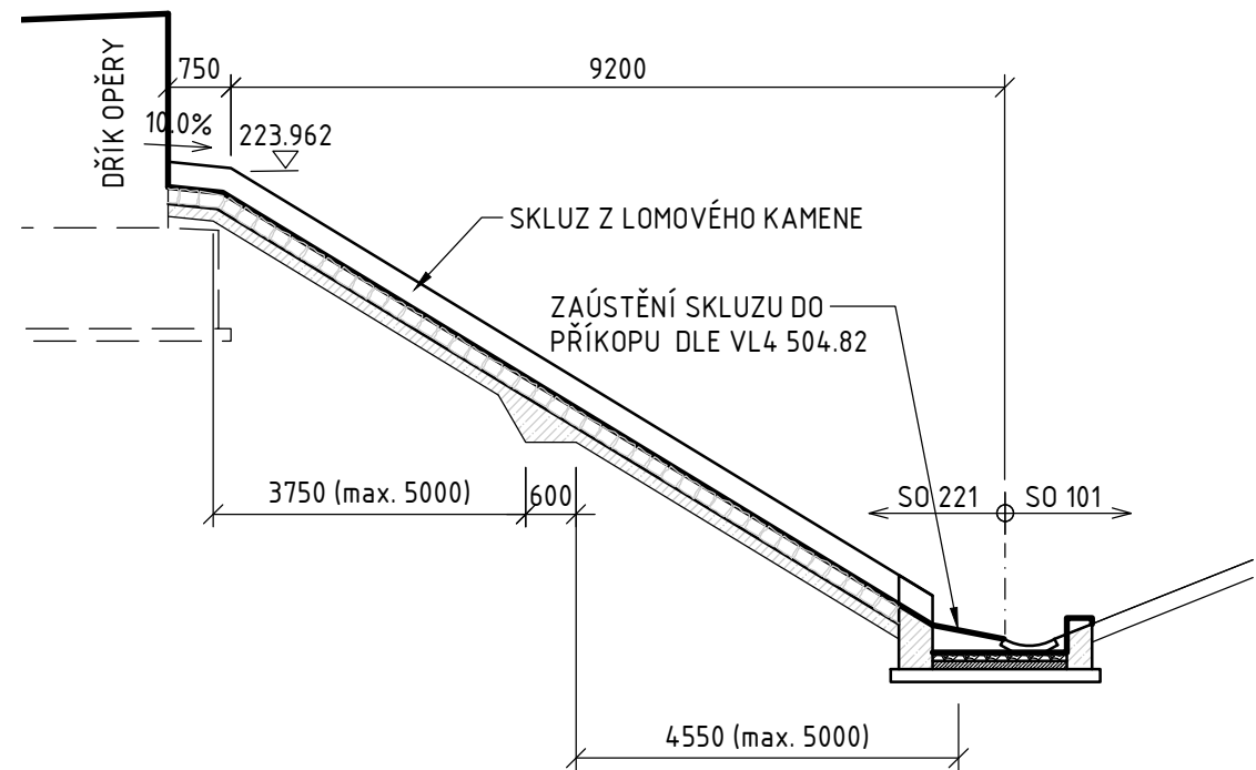
PODÉLNÝ ŘEZ SKLUZEM POD MOSTEM 1:100
