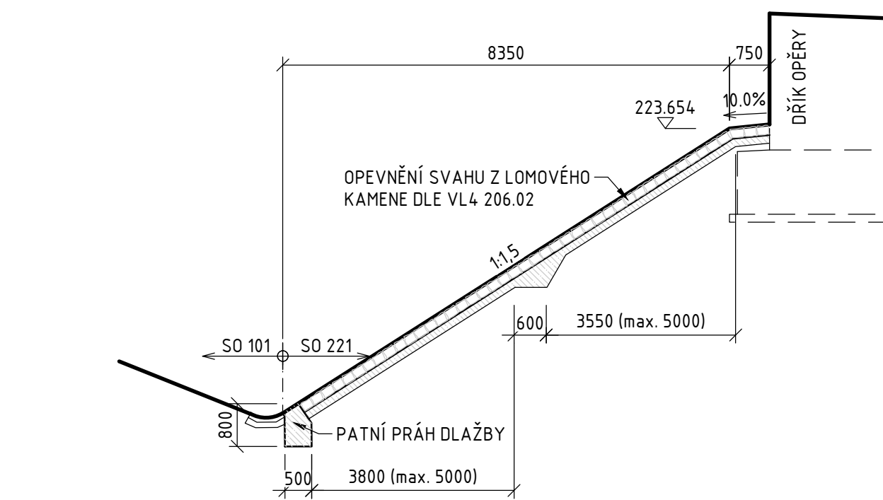
PODÉLNÝ ŘEZ ODLÁŽDĚNÍM POD MOSTEM 1:100
