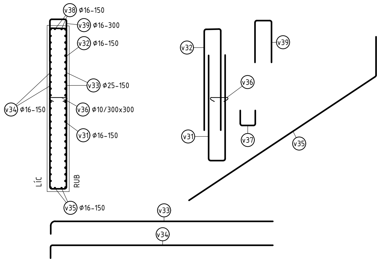
ŘEZ KŘÍDLEM 1:50
