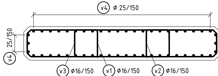
PŮDORYS DŘÍKU PILÍŘE 1:35
