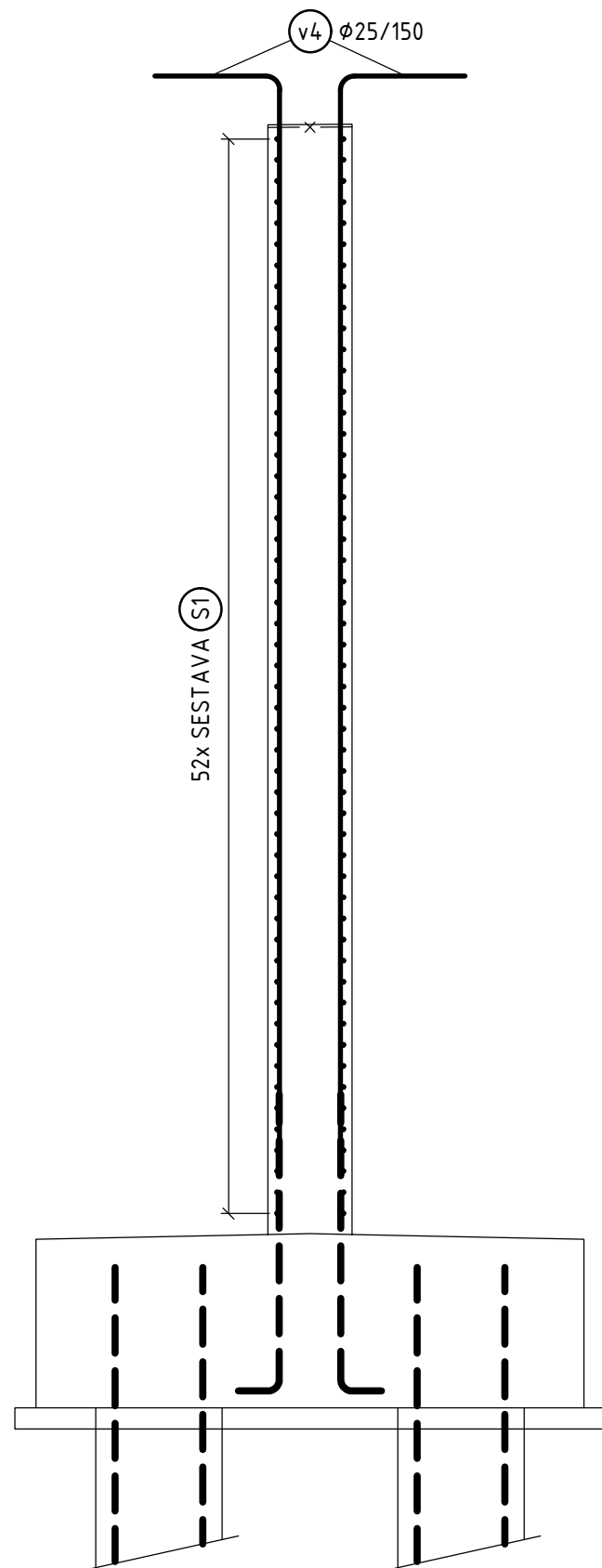
ŘEZ DŘÍKEM PILÍŘE 1:50
