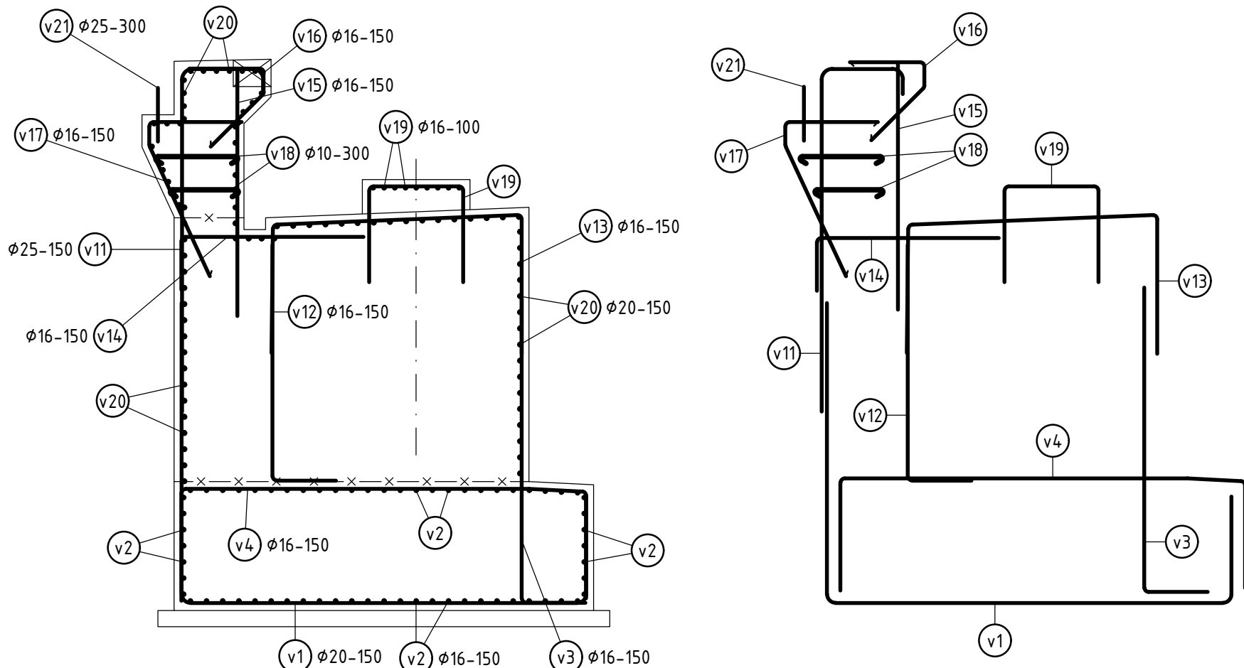
SCHÉMA VÝZTUŽE OPĚRY 01 PŘÍČNÝ ŘEZ 1:50
