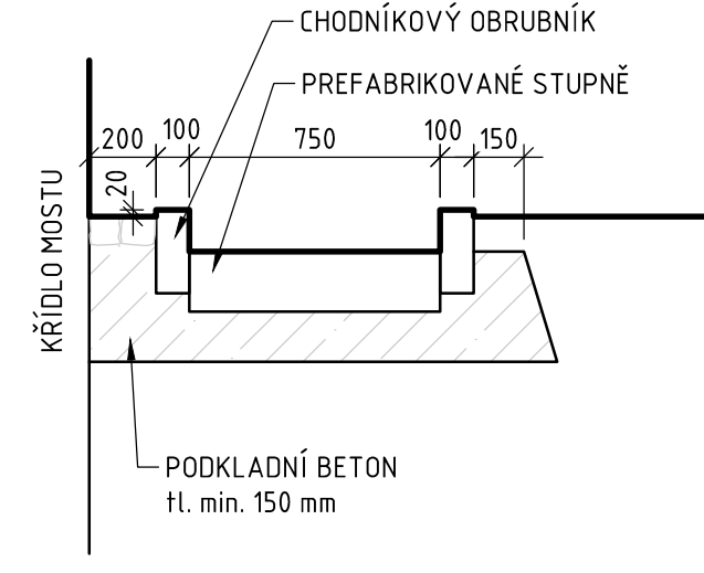
ŘEZ A-A 1:25
