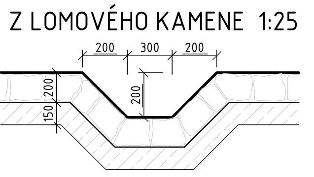
PŘÍČNÝ ŘEZ SKLUZEM
