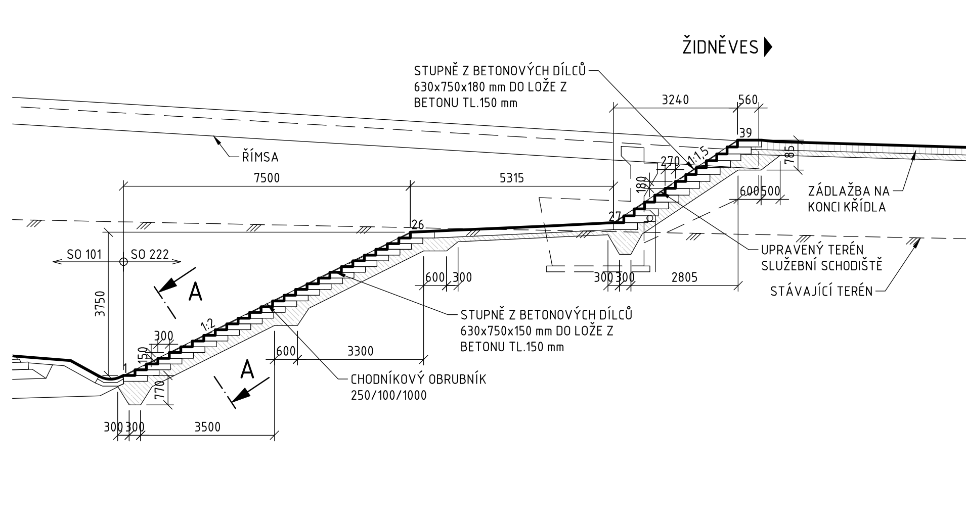
PODÉLNÝ ŘEZ ODLÁŽDĚNÍM POD MOSTEM 1:75
