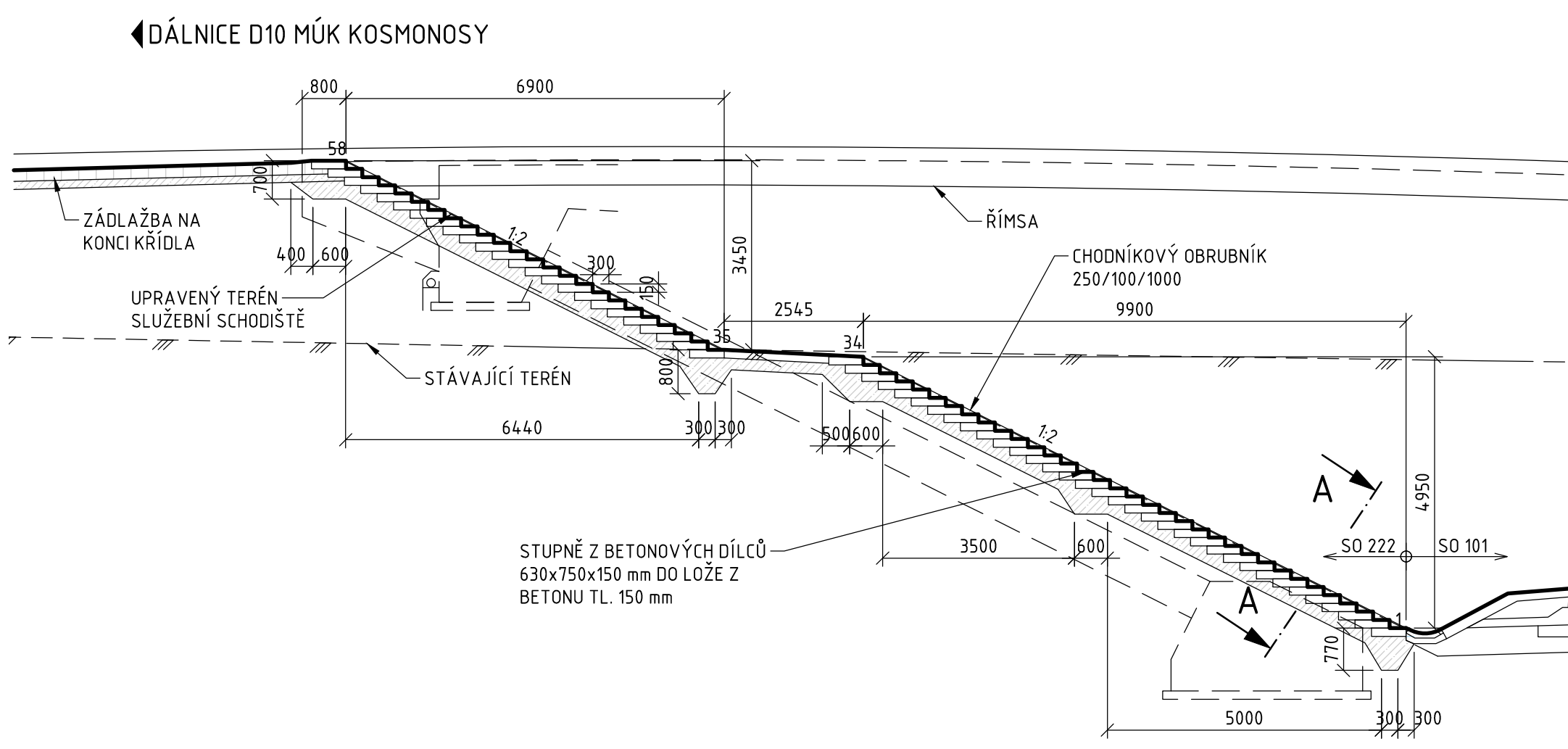
PODÉLNÝ ŘEZ ODLÁŽDĚNÍM POD MOSTEM 1:75
