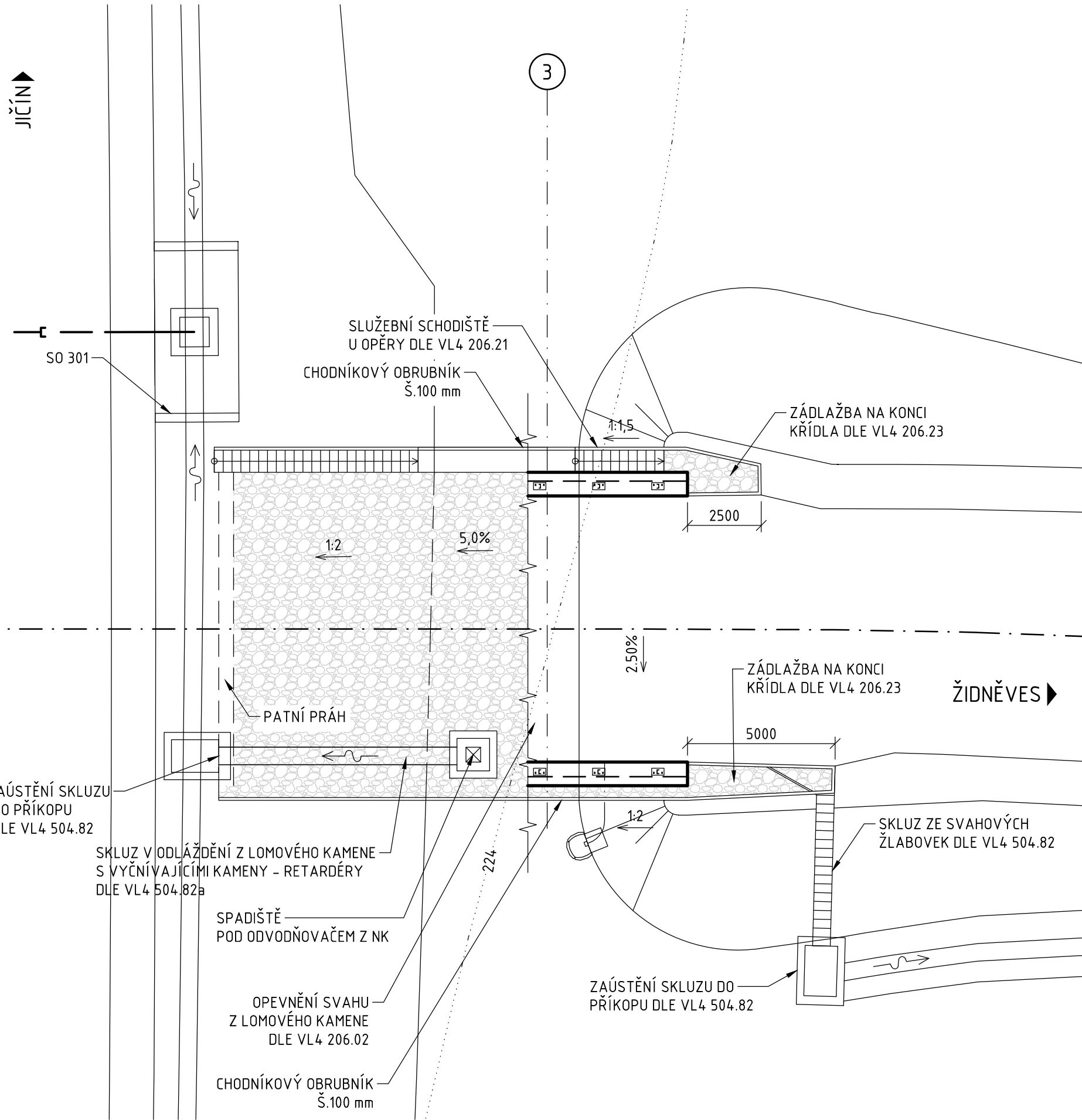
SLUŽEBNÍ SCHODIŠTĚ PODÉL KŘÍDLA OPĚRY 03 1: 100
