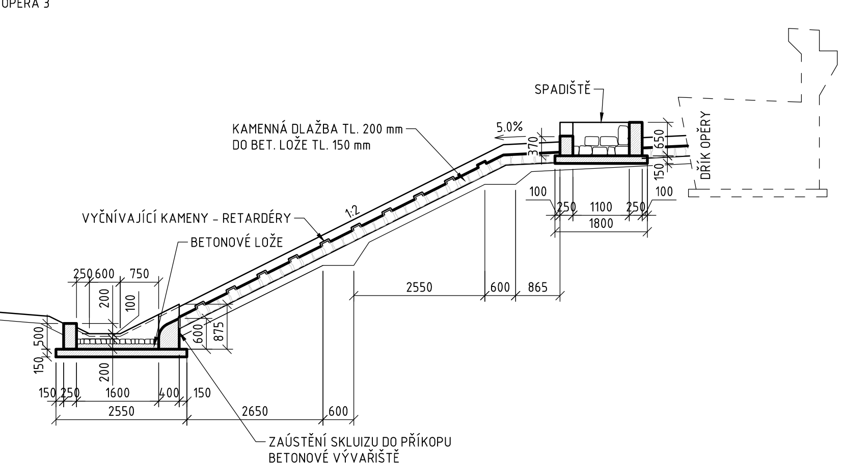
PODÉLNÝ ŘEZ SKLUZEM V ODLÁŽDĚNÍ POD MOSTEM 1:75
