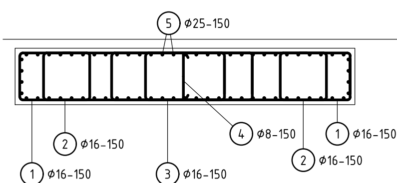
SCHÉMA VÝZTUŽE PODPĚRY P2 - PŘEDNÍ VZPĚRA PŘÍČNÝ ŘEZ 1:50
