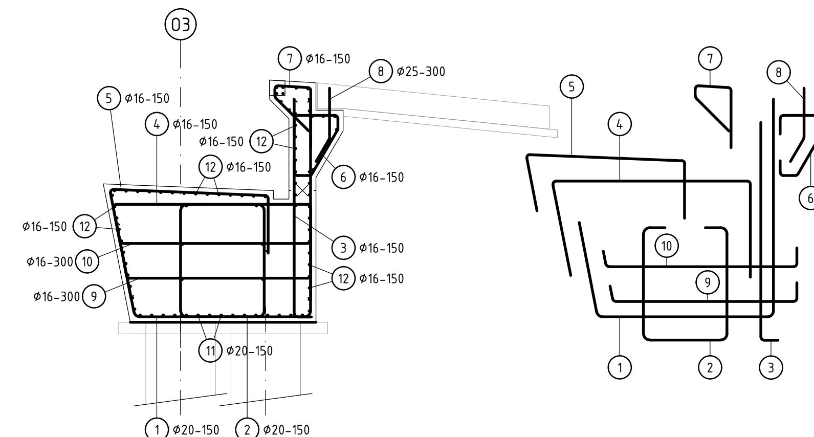
SCHÉMA VÝZTUŽE OPĚRY 03 PŘÍČNÝ ŘEZ 1:50
