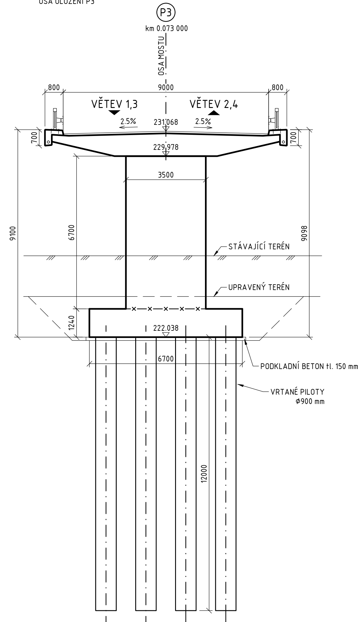
ŘEZ C-C 1:100 OSA ULOŽENÍ P3
