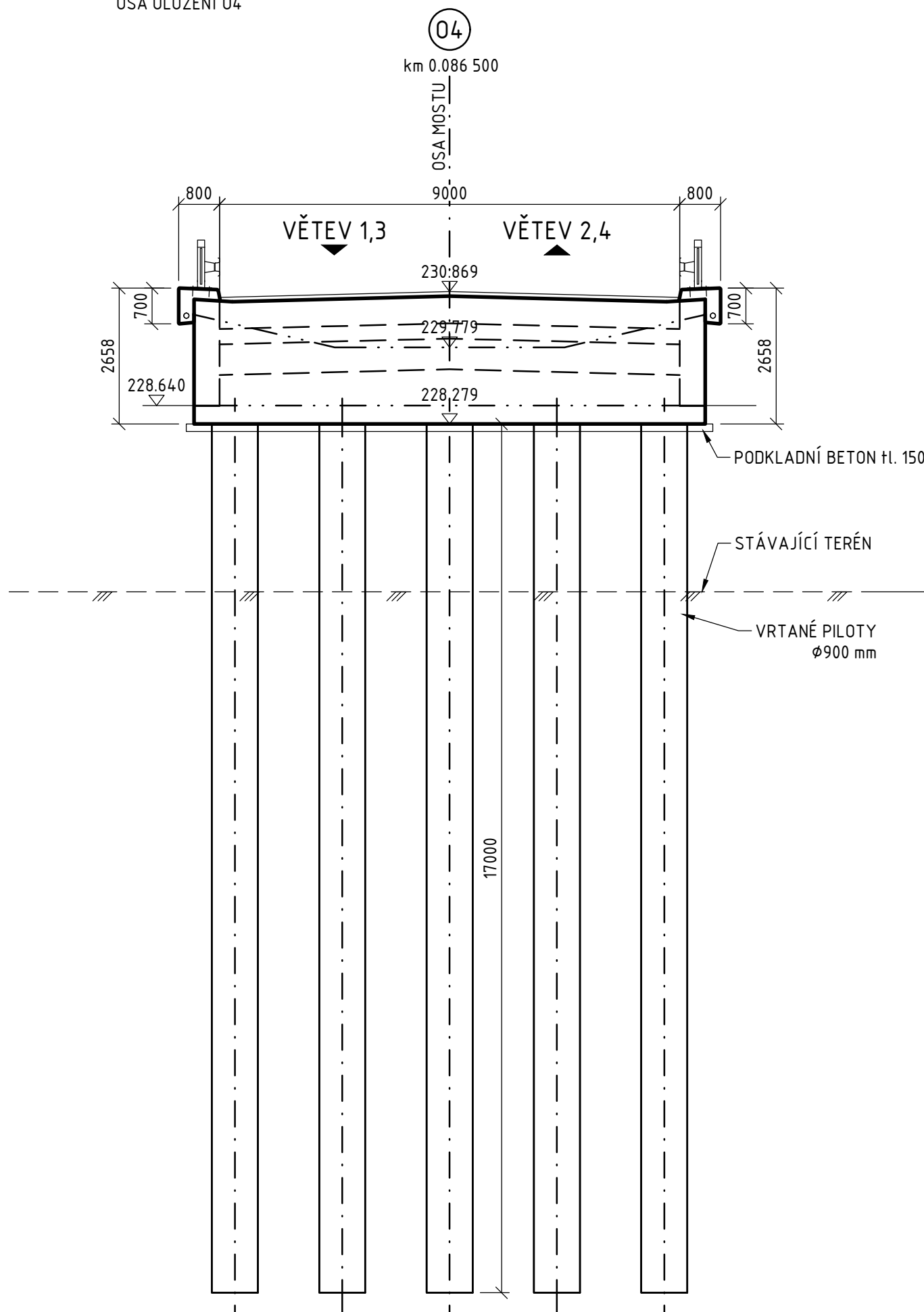
ŘEZ D-D 1:100 OSA ULOŽENÍ 04
