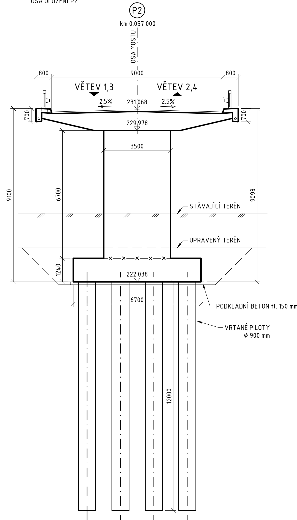
ŘEZ B-B 1:100 OSA ULOŽENÍ P2
