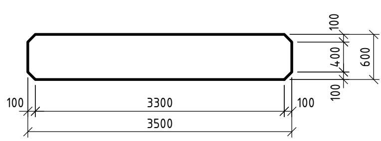
ŘEZ STOJKOU 1:50
