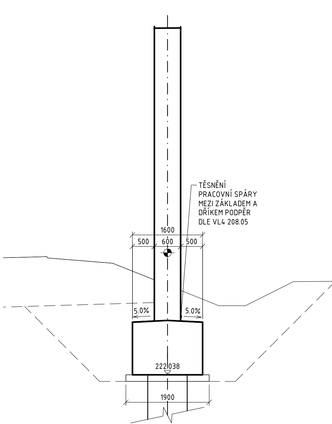
ŘEZ D-D 1:50
