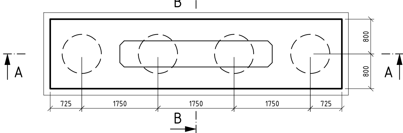
PŮDORYS ZÁKLADU 1:50
