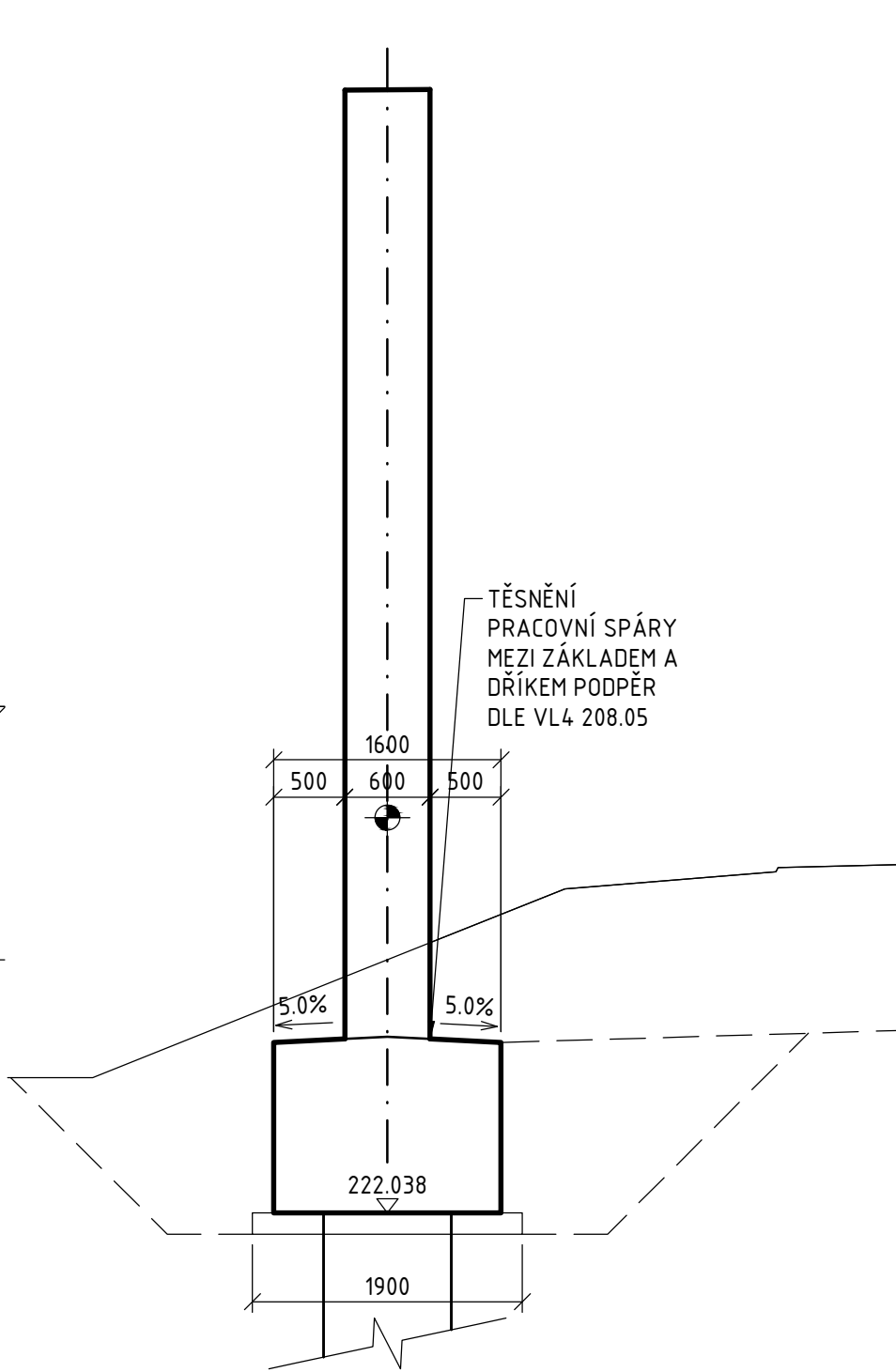
ŘEZ B-B 1:50
