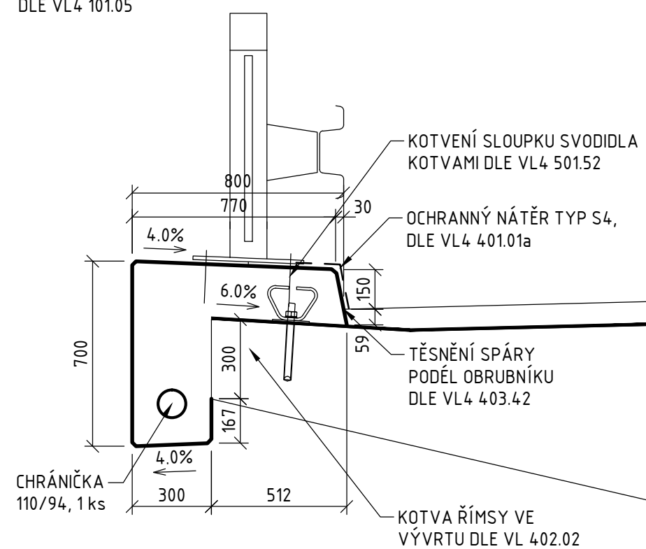
ŘEZ A-A 1:20
