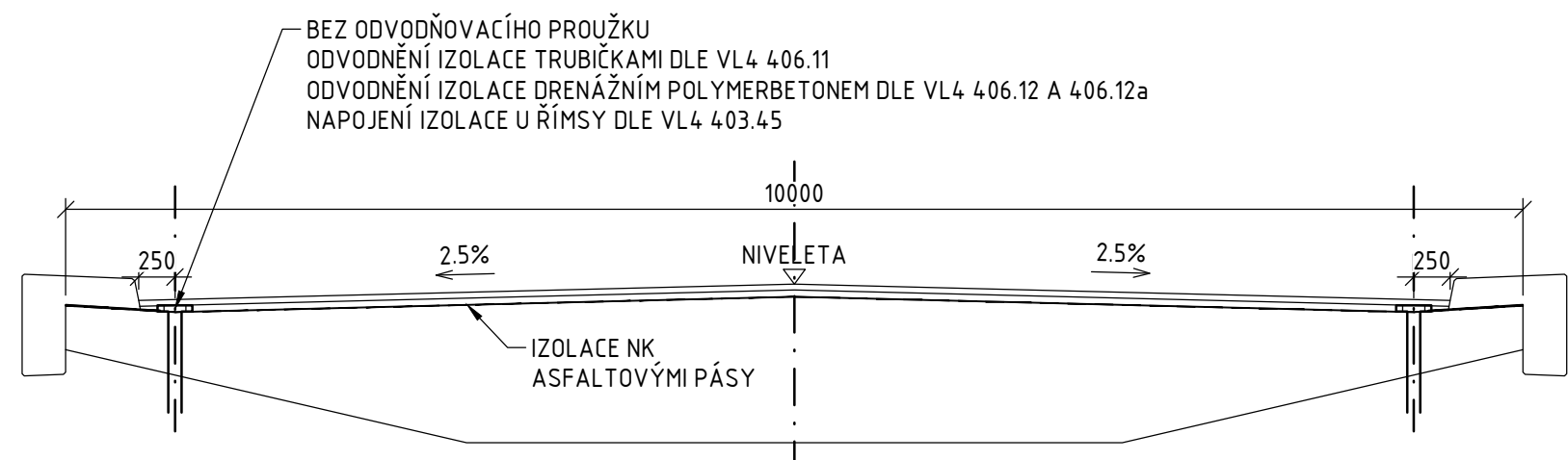
PŘÍČNÝ ŘEZ 1:50
