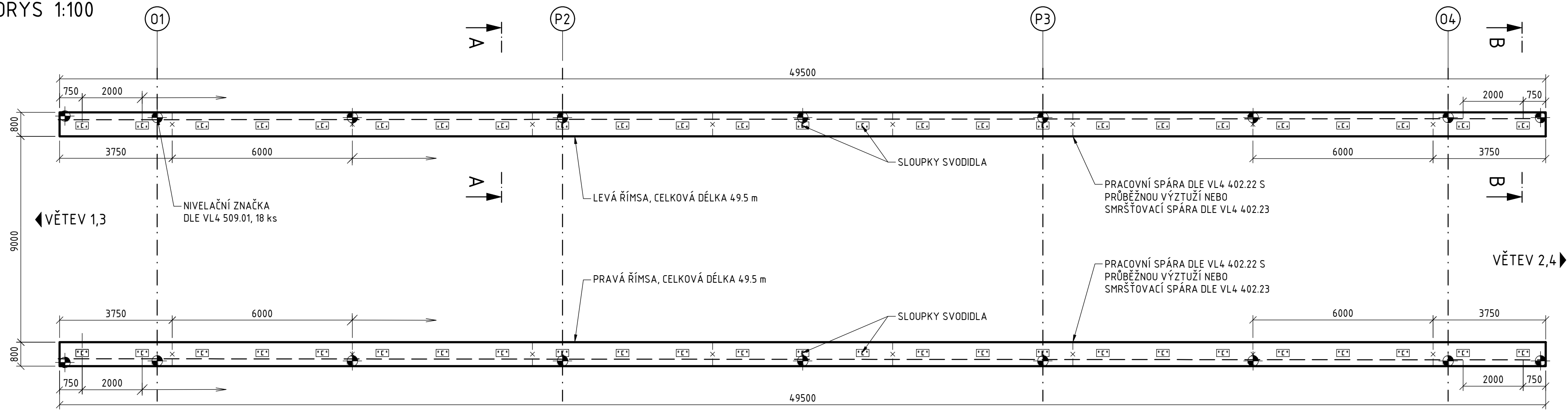
PŮDORYS 1:100
