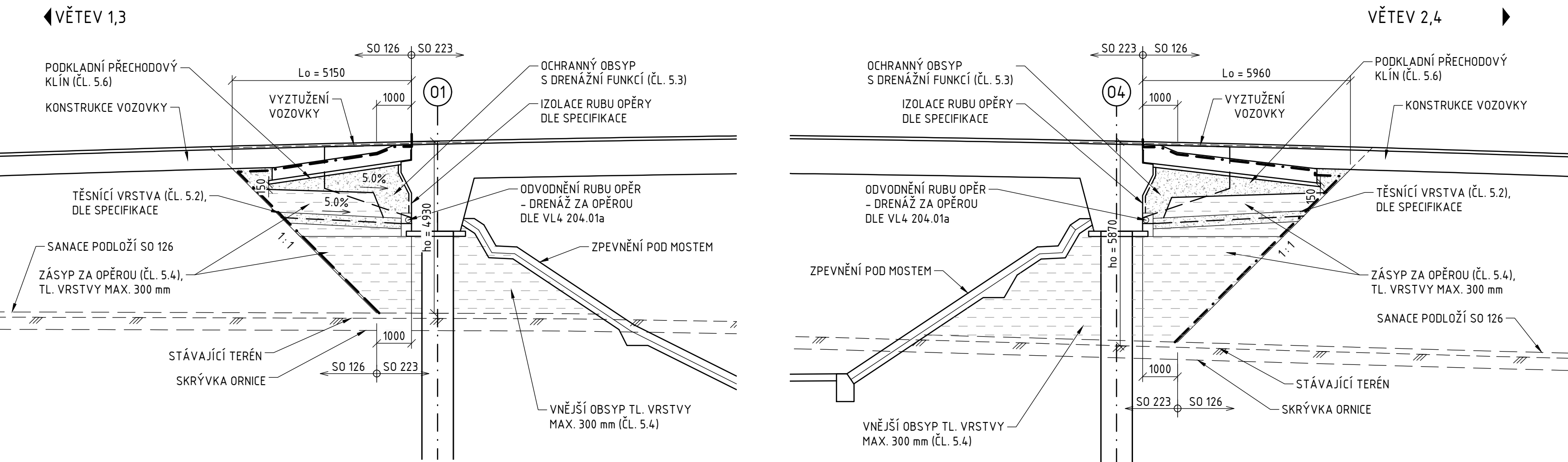
PŘECHODOVÉ OBLASTI, PODÉLNÝ ŘEZ 1:100
