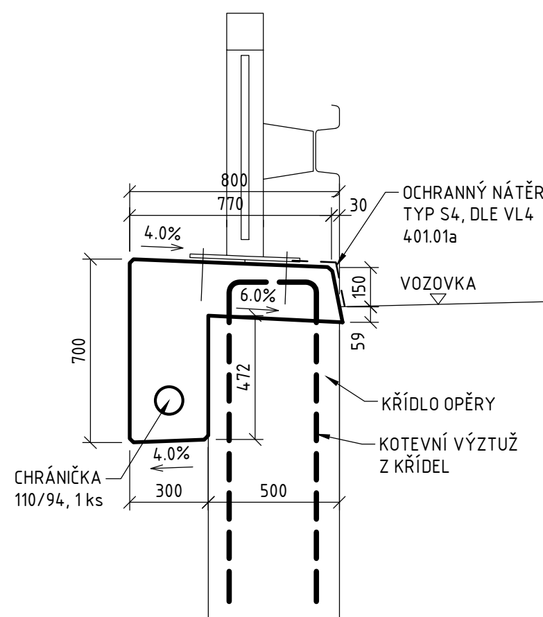
ŘEZ B-B 1:20
