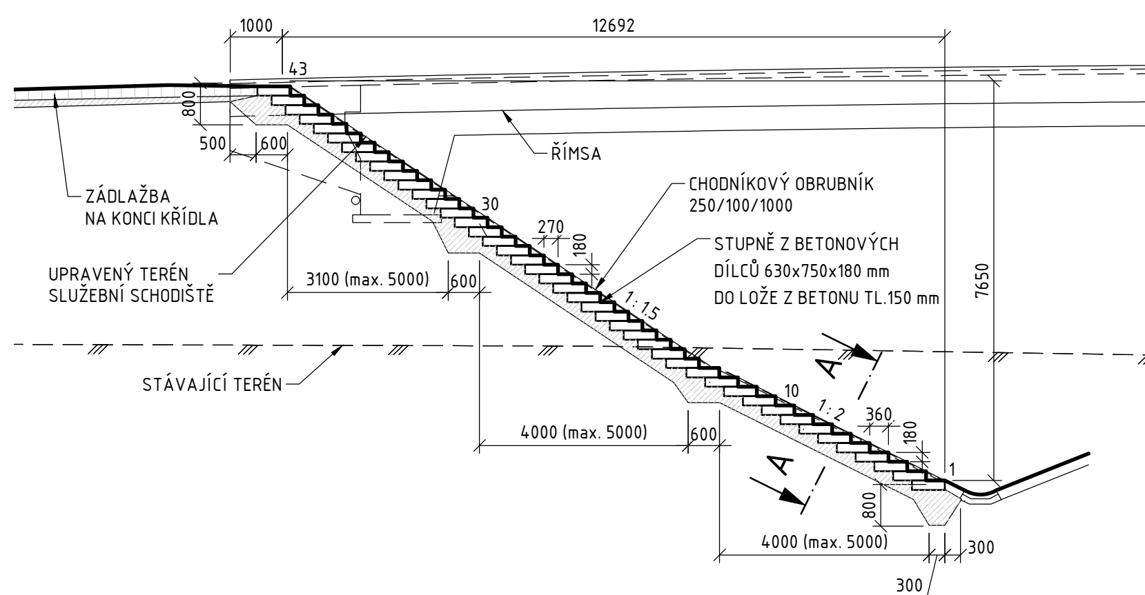
SLUŽEBNÍ SCHODIŠTĚ PODÉL KŘÍDLA OPĚRY 01 1: 100 VĚTEV 1,3
