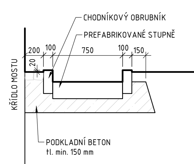
ŘEZ A-A 1:25
