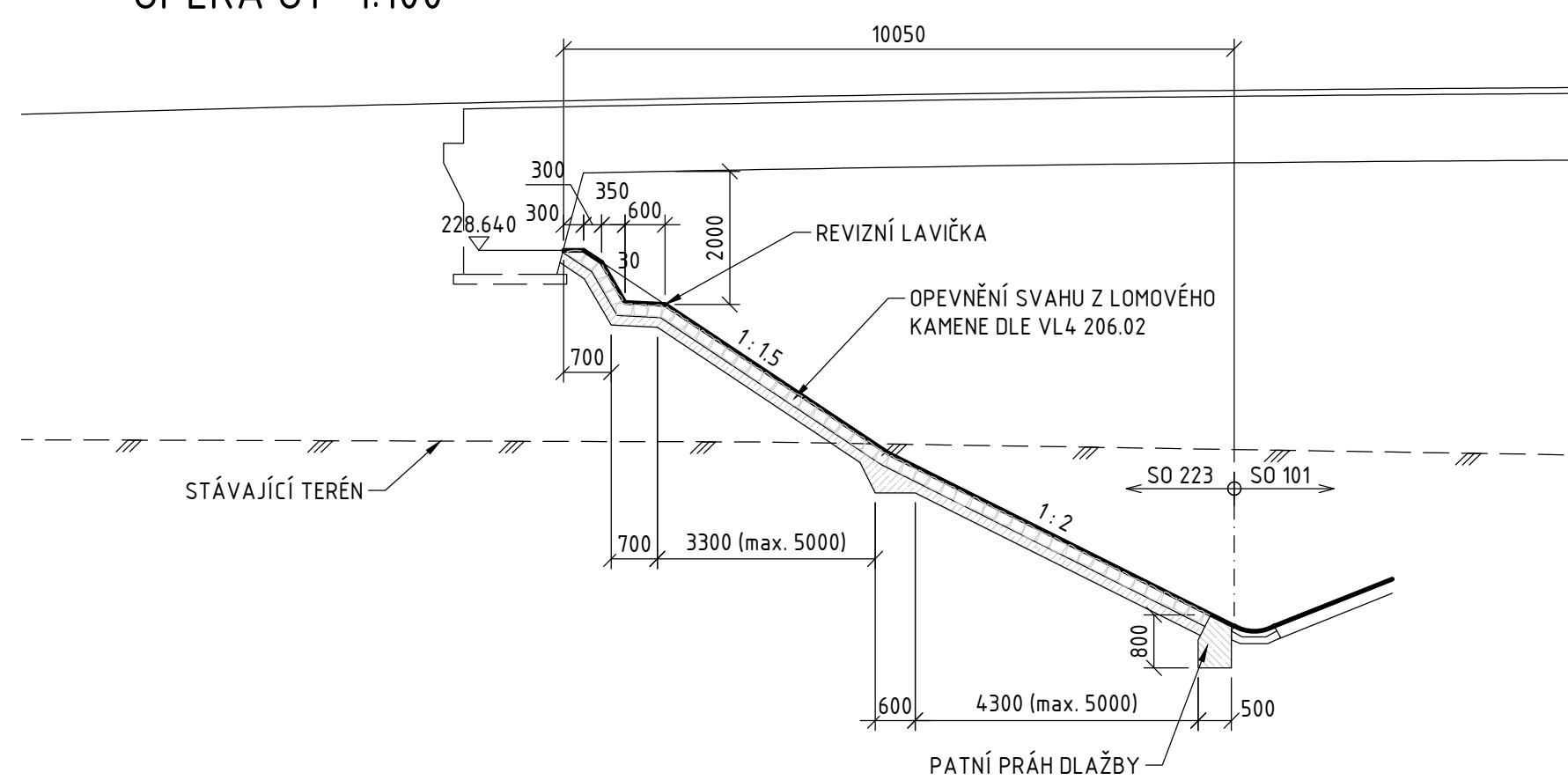
PODÉLNÝ ŘEZ ODLÁŽDĚNÍM POD MOSTEM OPĚRA 01 1:100
