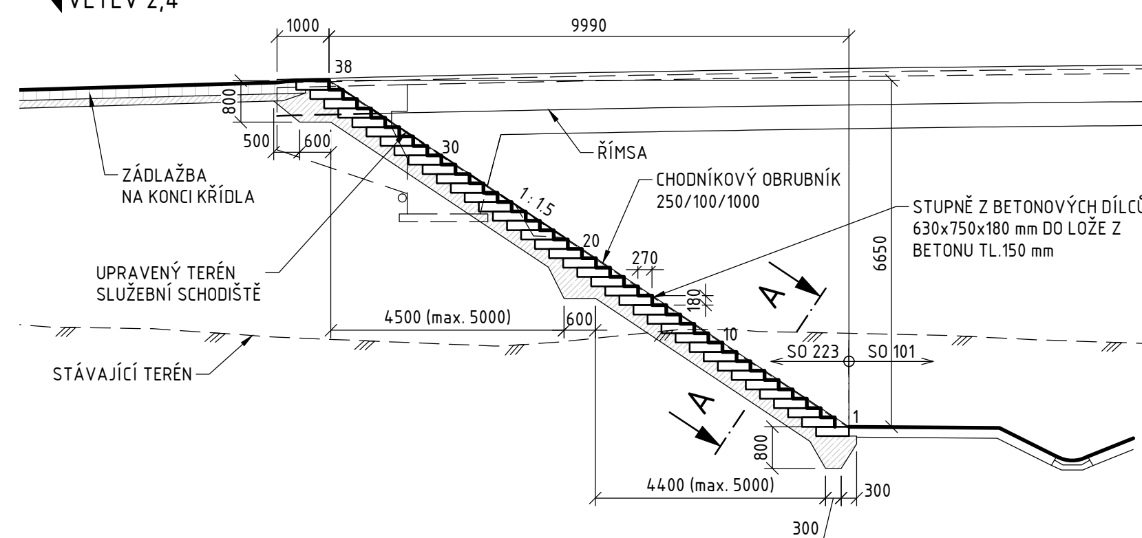
SLUŽEBNÍ SCHODIŠTĚ PODÉL KŘÍDLA OPĚRY 04 1: 100 VĚTEV 2,4
