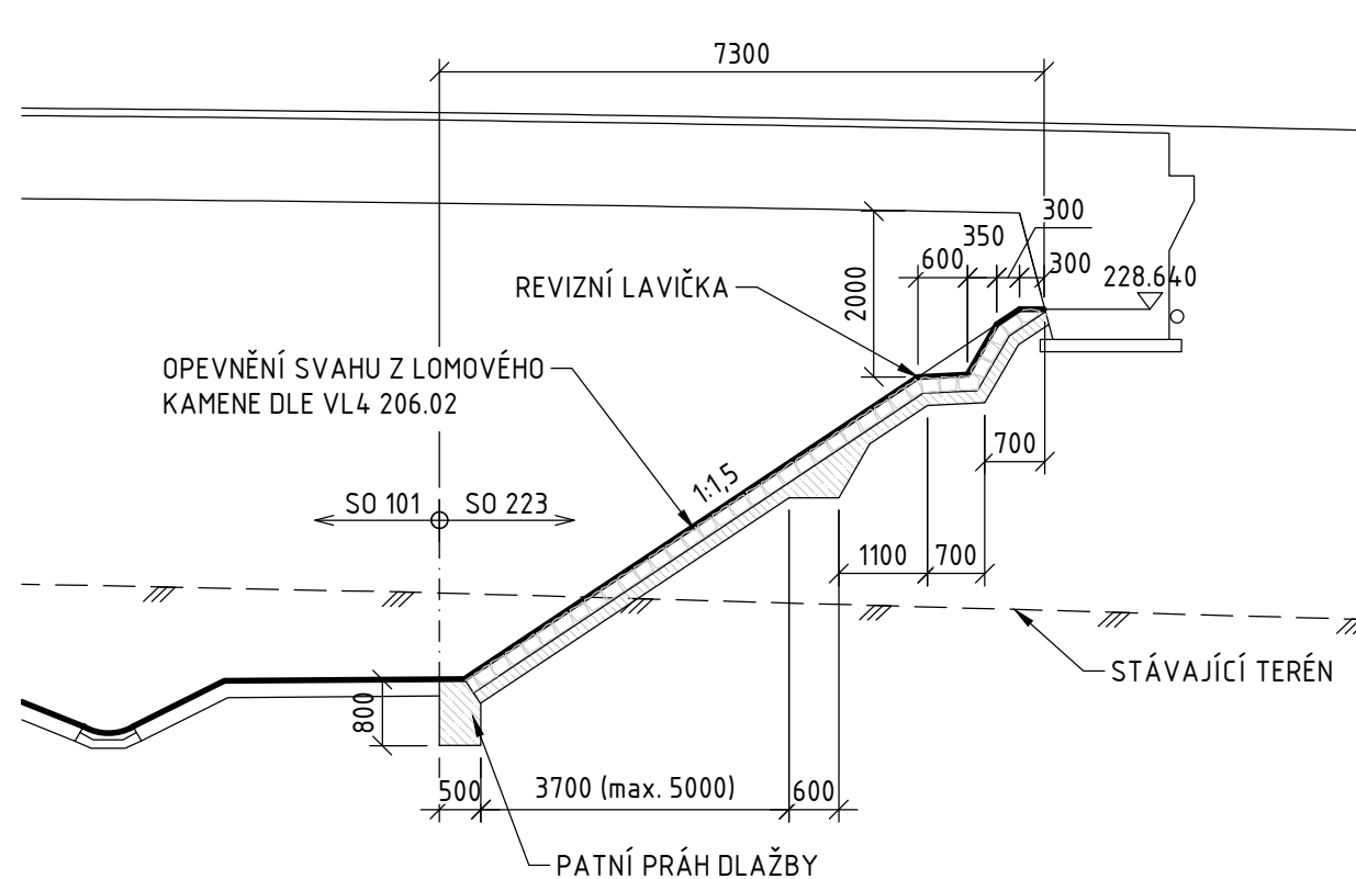
PODÉLNÝ ŘEZ ODLÁŽDĚNÍM POD MOSTEM OPĚRA 04 1:100
