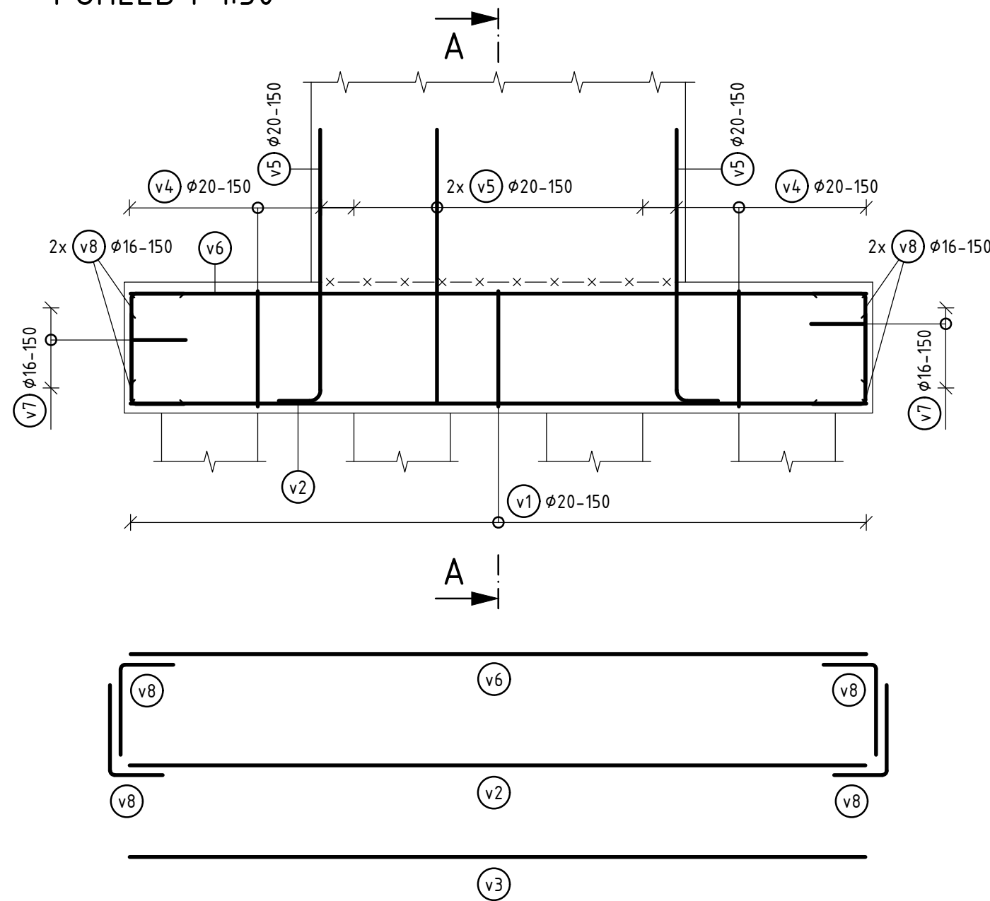
POHLED 1 1:50
