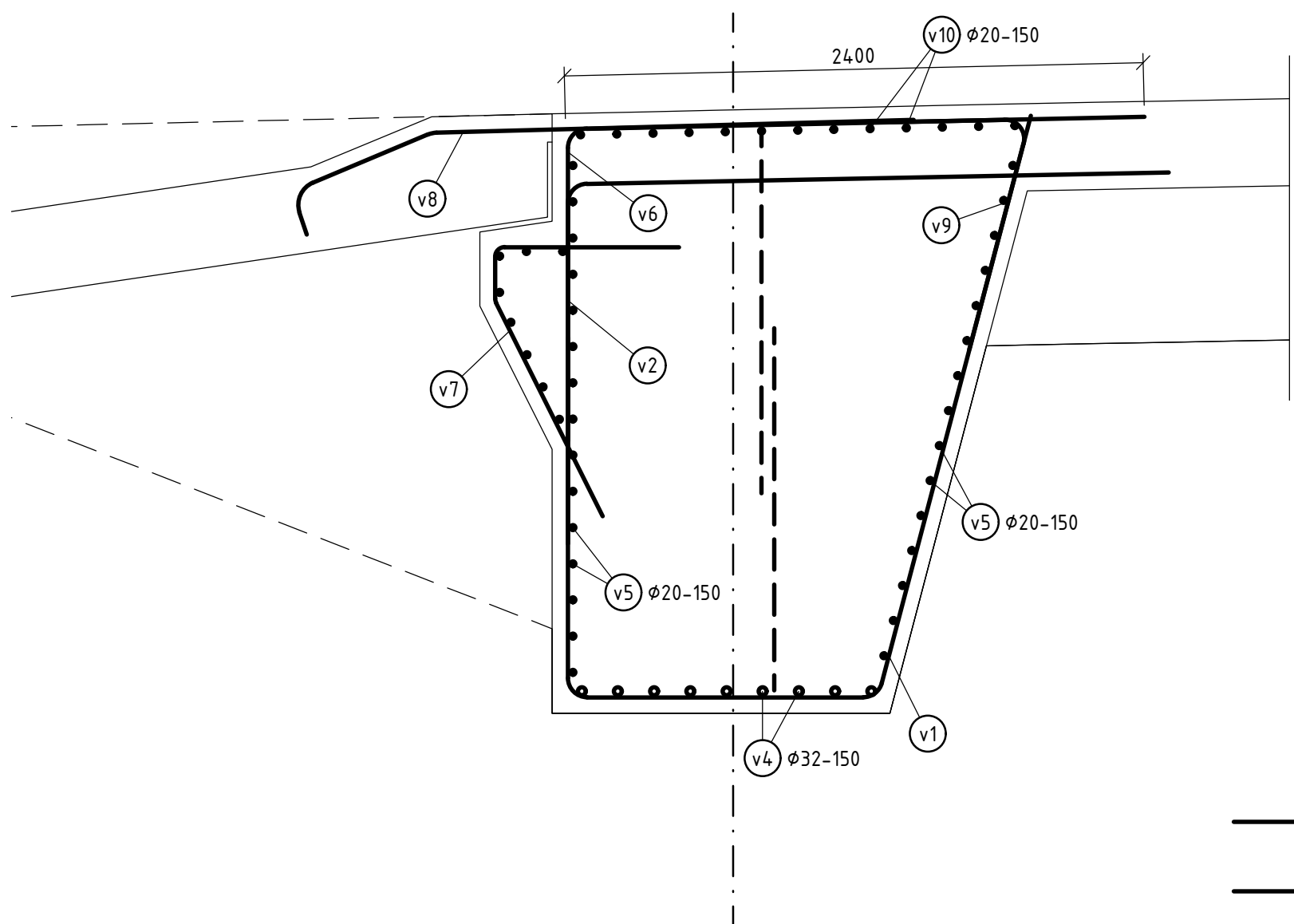
SCHÉMA VÝZTUŽE NOSNÉ KONSTRUKCE PŘÍČNÝ ŘEZ 1:25 V KRAJNÍM PŘÍČNÍKU
