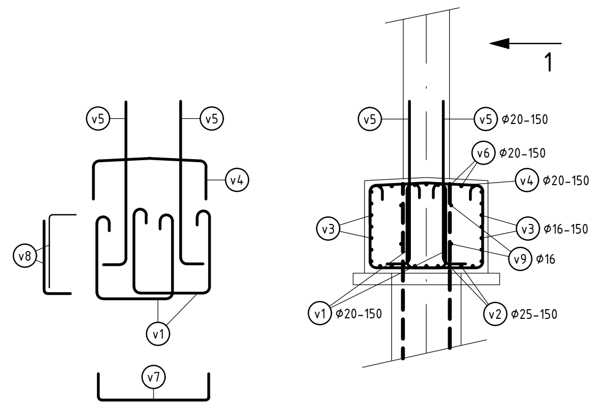
SCHÉMA VÝZTUŽE ZÁKLADŮ PILÍŘŮ PŘÍČNÝ ŘEZ A-A 1:50
