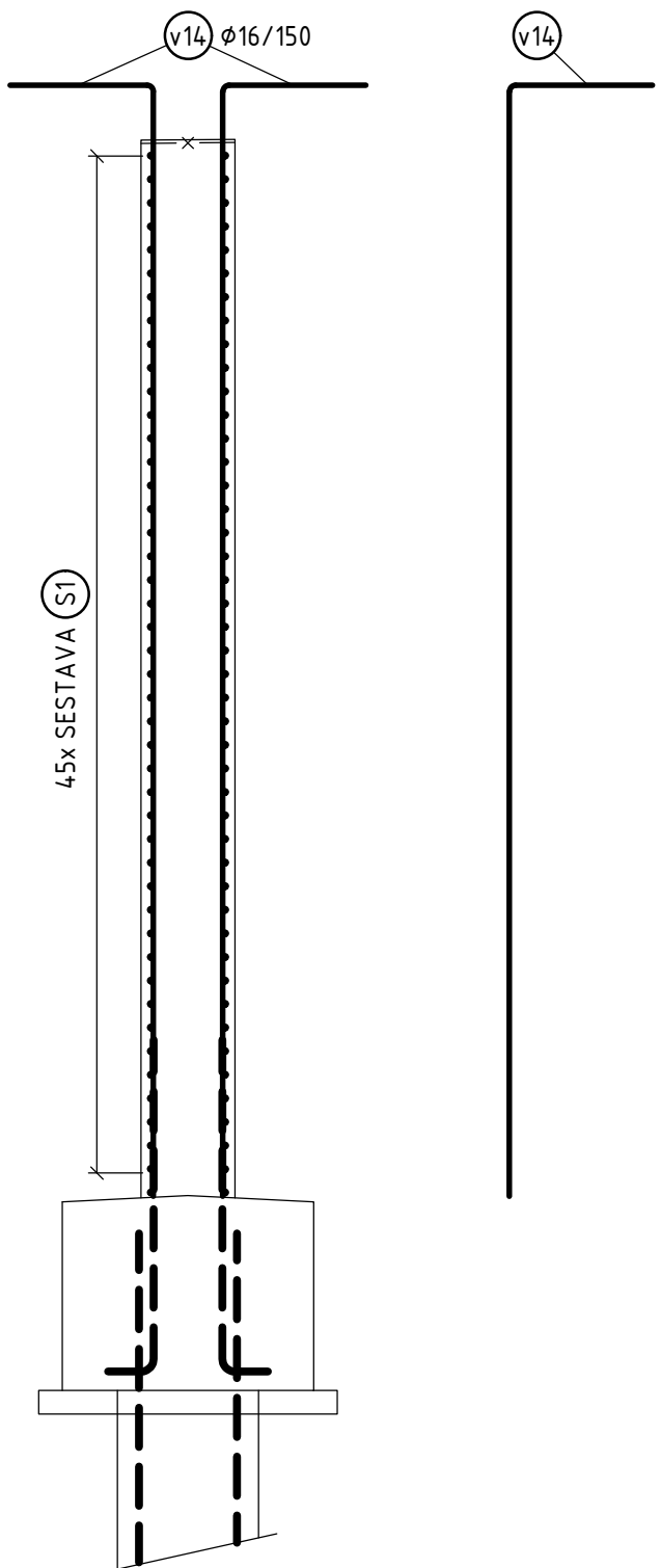
ŘEZ DŘÍKEM PILÍŘE 1:50
