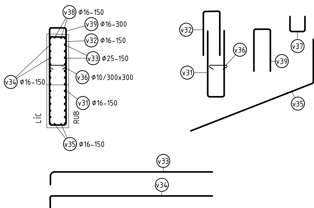
ŘEZ KŘÍDLEM 1:50
