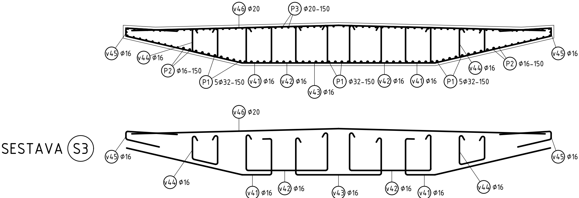
SCHÉMA VÝZTUŽE NOSNÉ KONSTRUKCE PŘÍČNÝ ŘEZ V POLI 1:50
