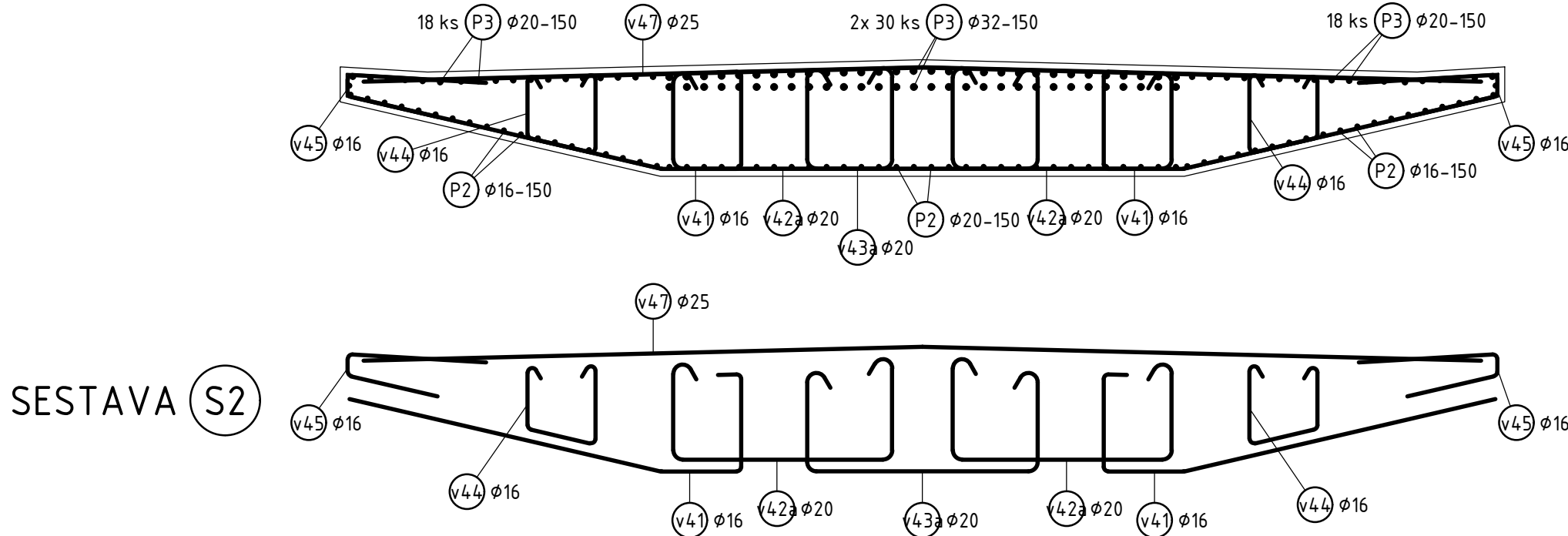
SCHÉMA VÝZTUŽE NOSNÉ KONSTRUKCE PŘÍČNÝ ŘEZ NAD PODPOROU 1:50
