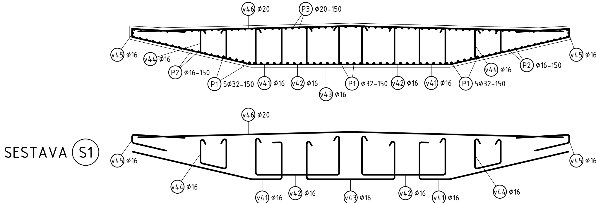
SCHÉMA VÝZTUŽE NOSNÉ KONSTRUKCE PŘÍČNÝ ŘEZ PŘED OPĚROU 1:50
