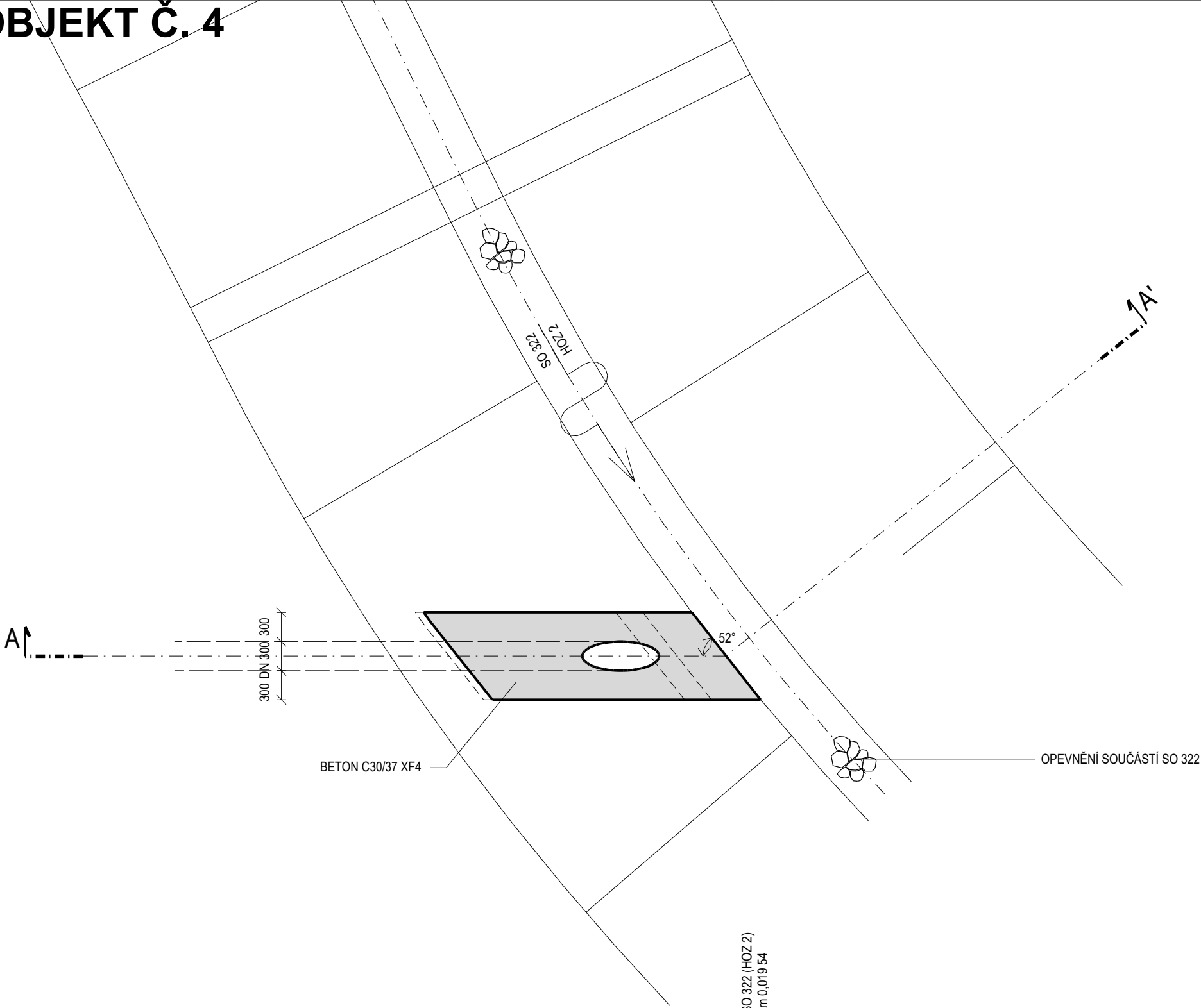
PŮDORYS
