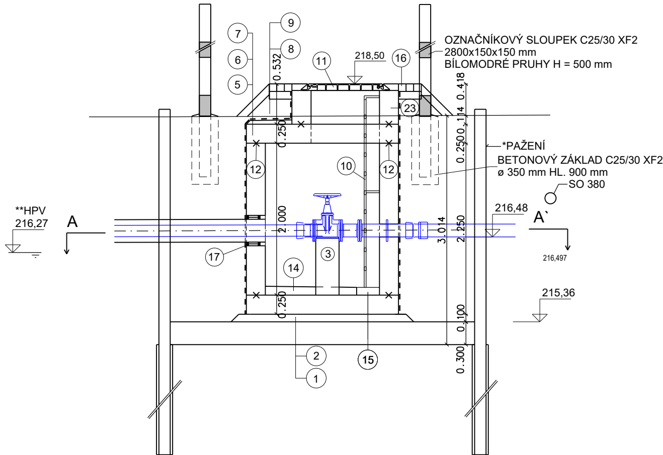
ŘEZ B - B'
