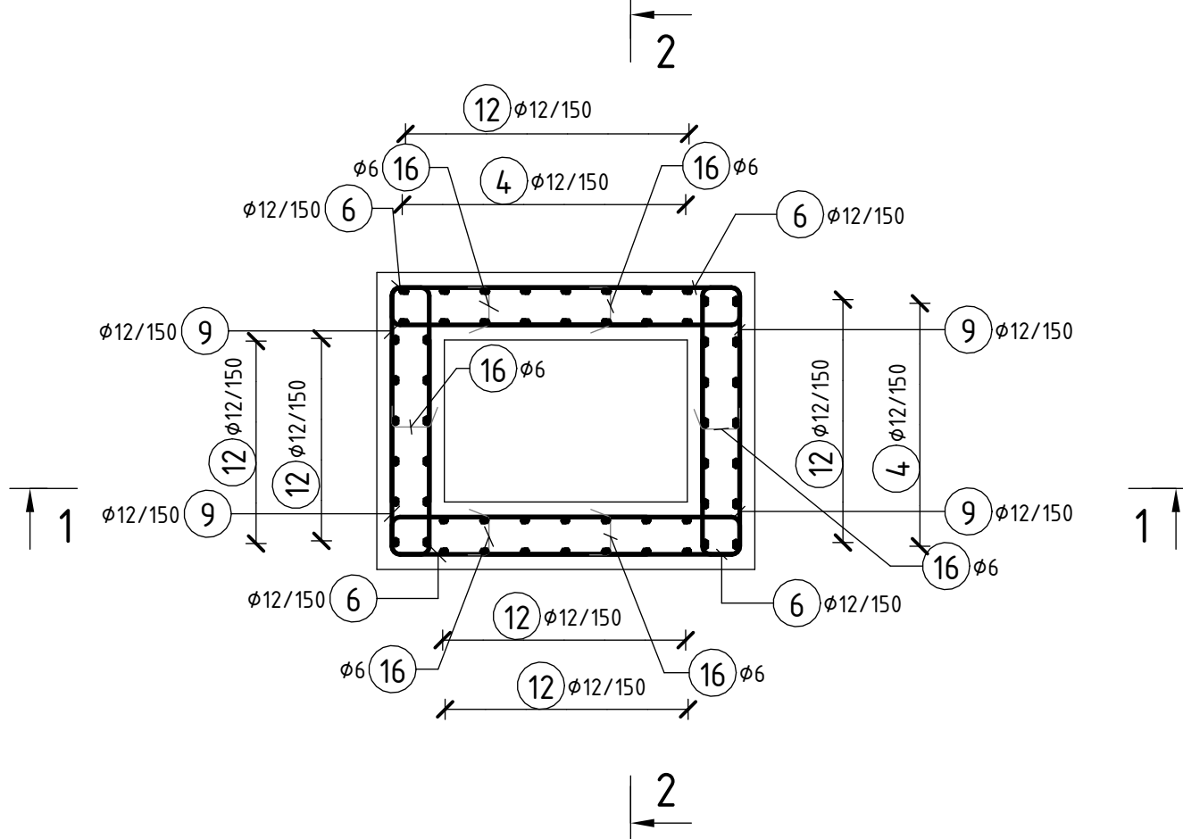
ŘEZ 4-4 1: 25
