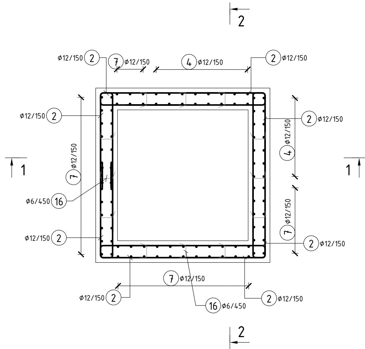
ŘEZ 3-3 1: 25
