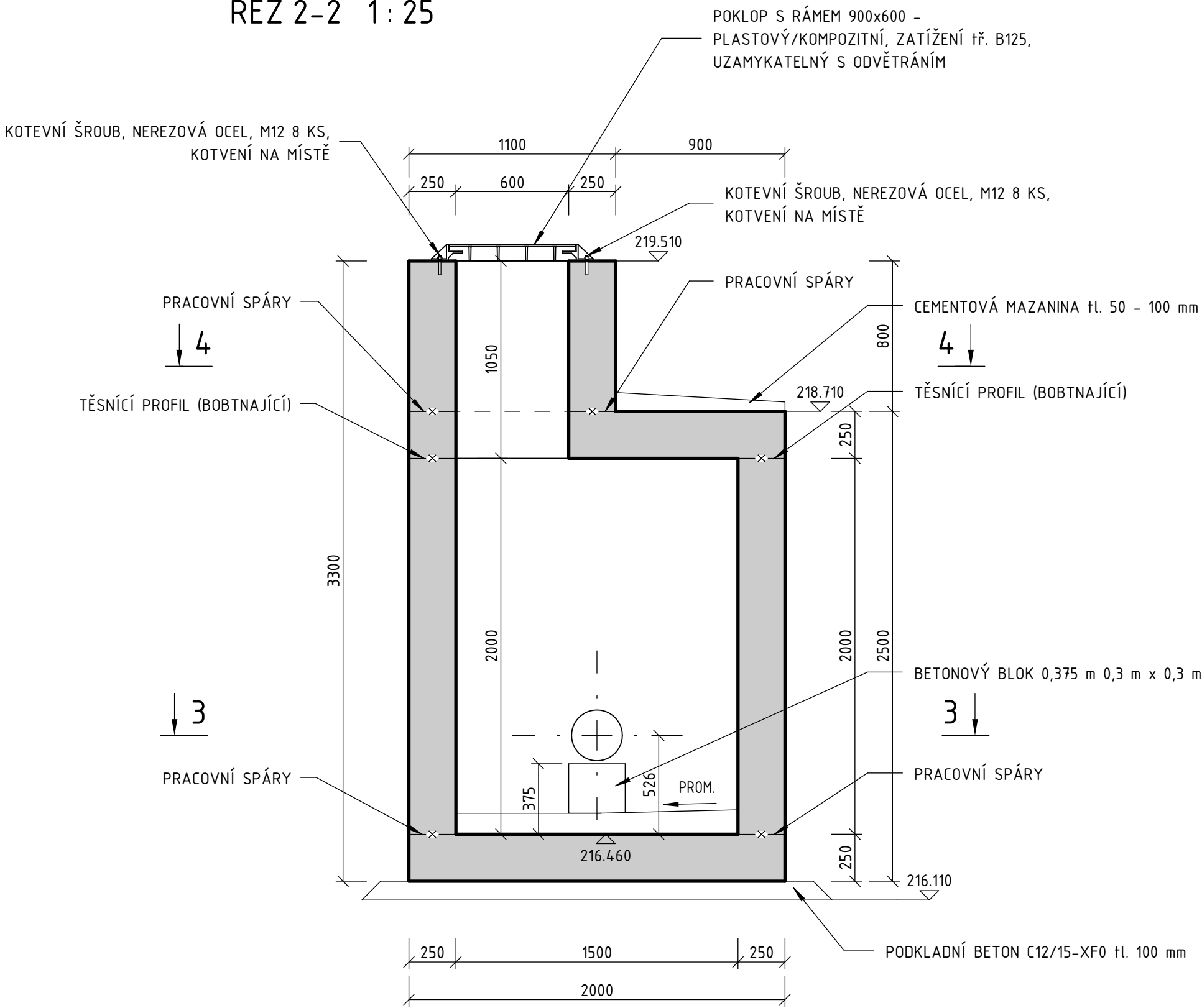
ŘEZ 2-2 1:25
