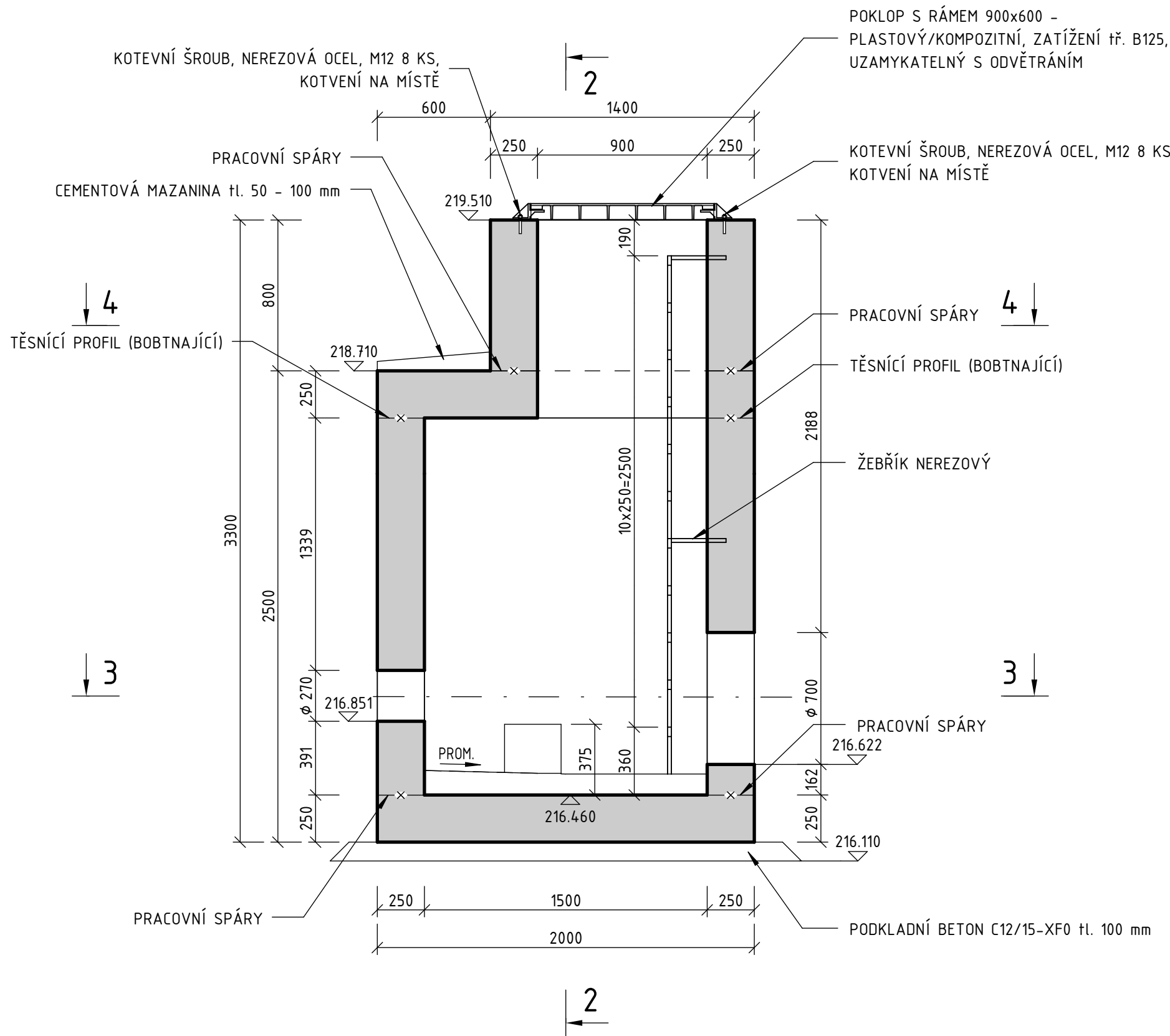
ŘEZ 1-1 1:25
