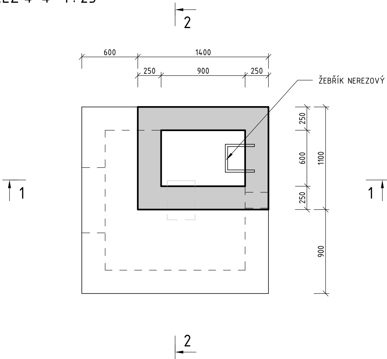
ŘEZ 4-4 1: 25
