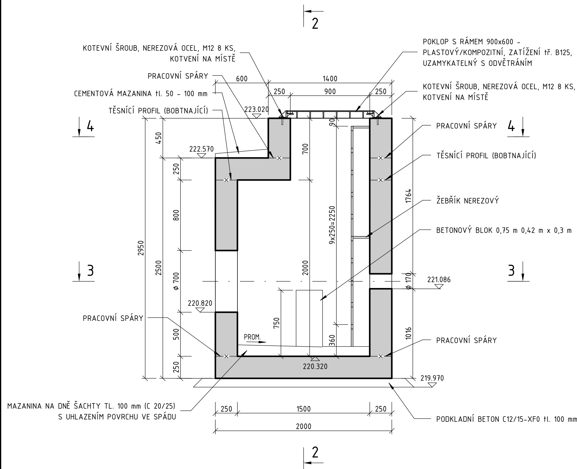
ŘEZ 1-1 1: 25
