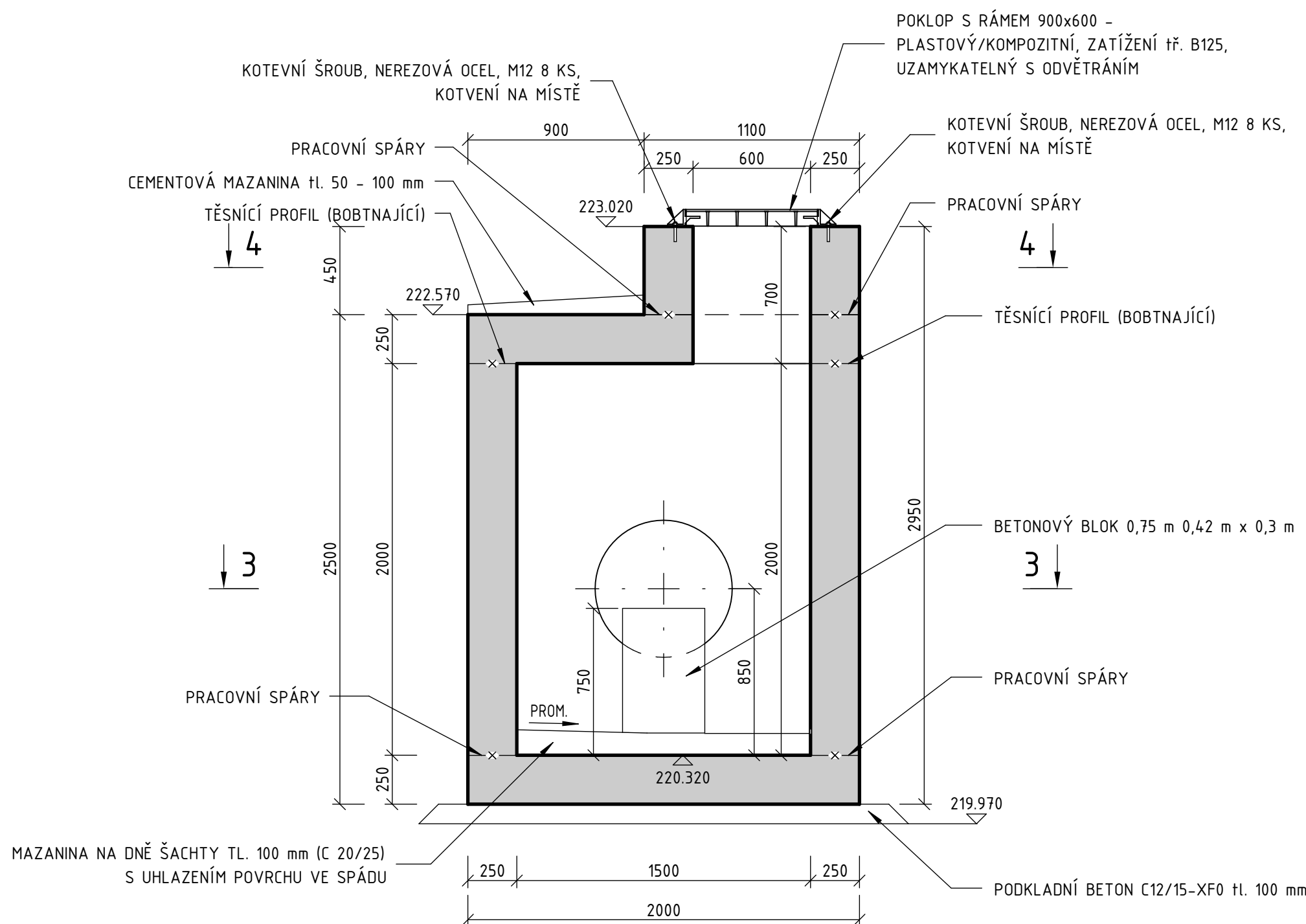
ŘEZ 2-2 1: 25
