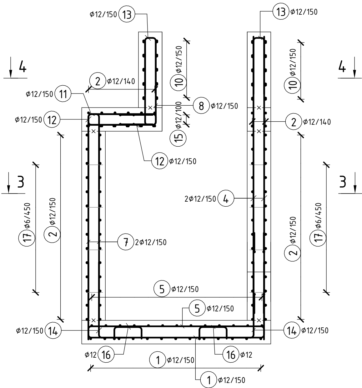
ŘEZ 1-1 1: 25
