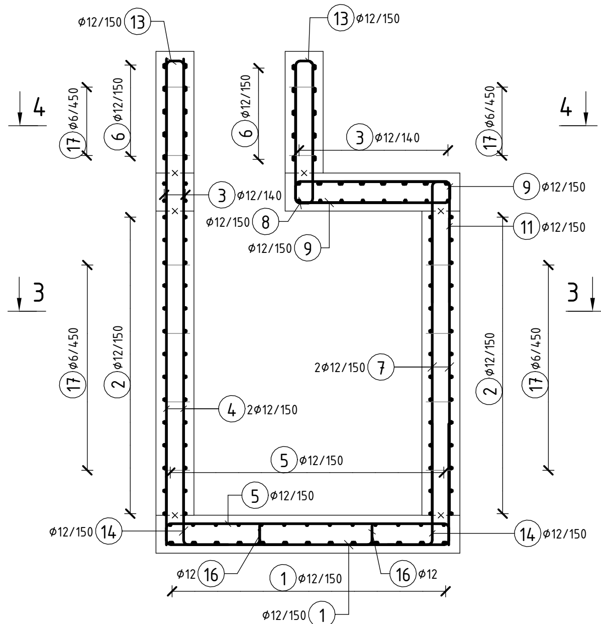
ŘEZ 2-2 1: 25
