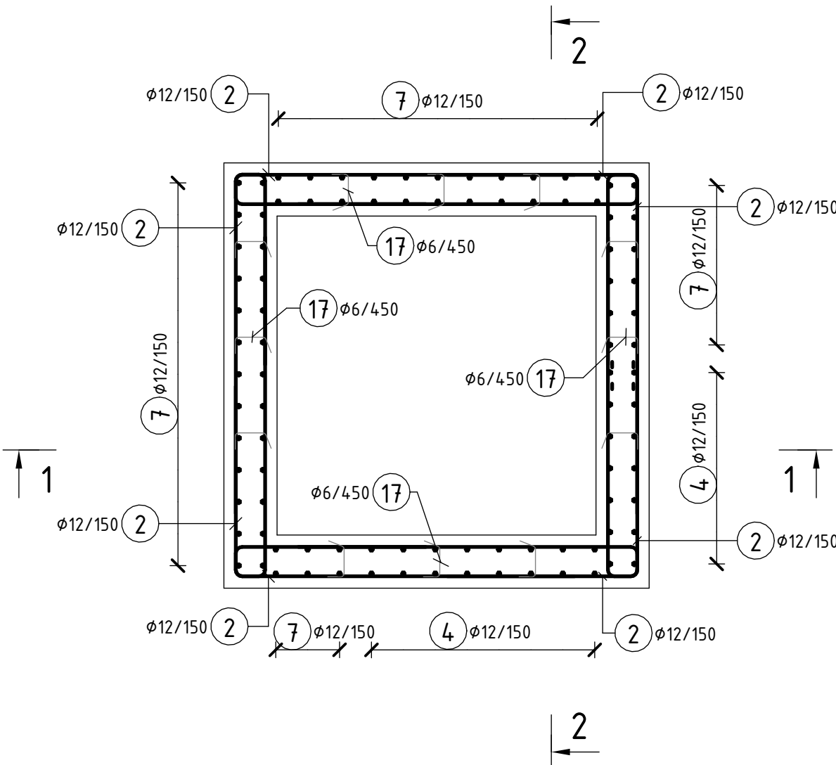
ŘEZ 3-3 1: 25
