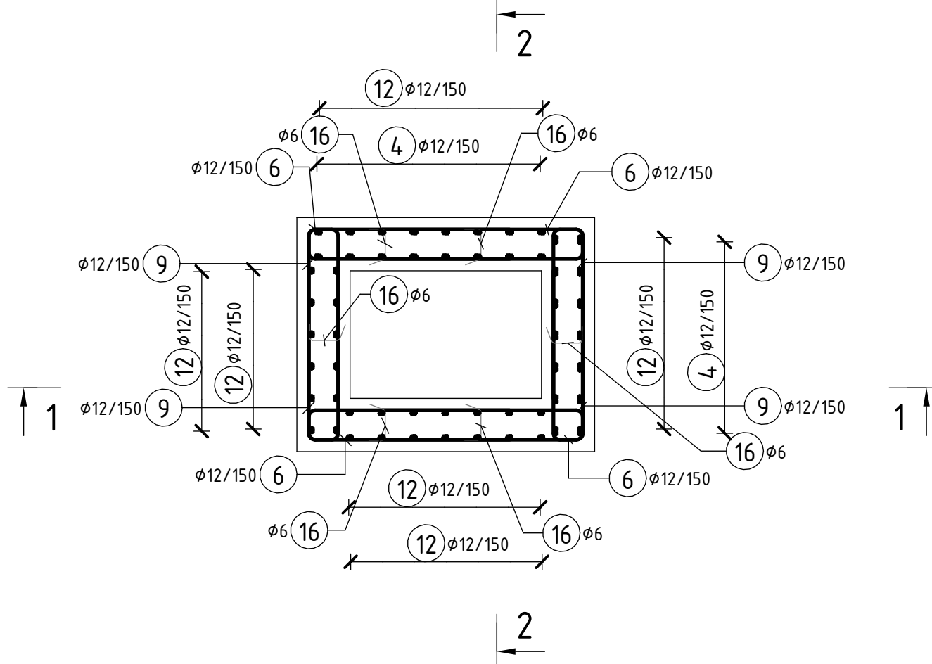
ŘEZ 4-4 1: 25
