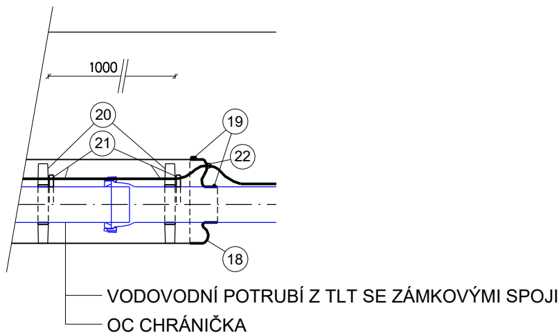
VZOROVÝ PODÉLNÝ ŘEZ CHRÁNIČKOU S POTRUBÍM M 1 : 25
