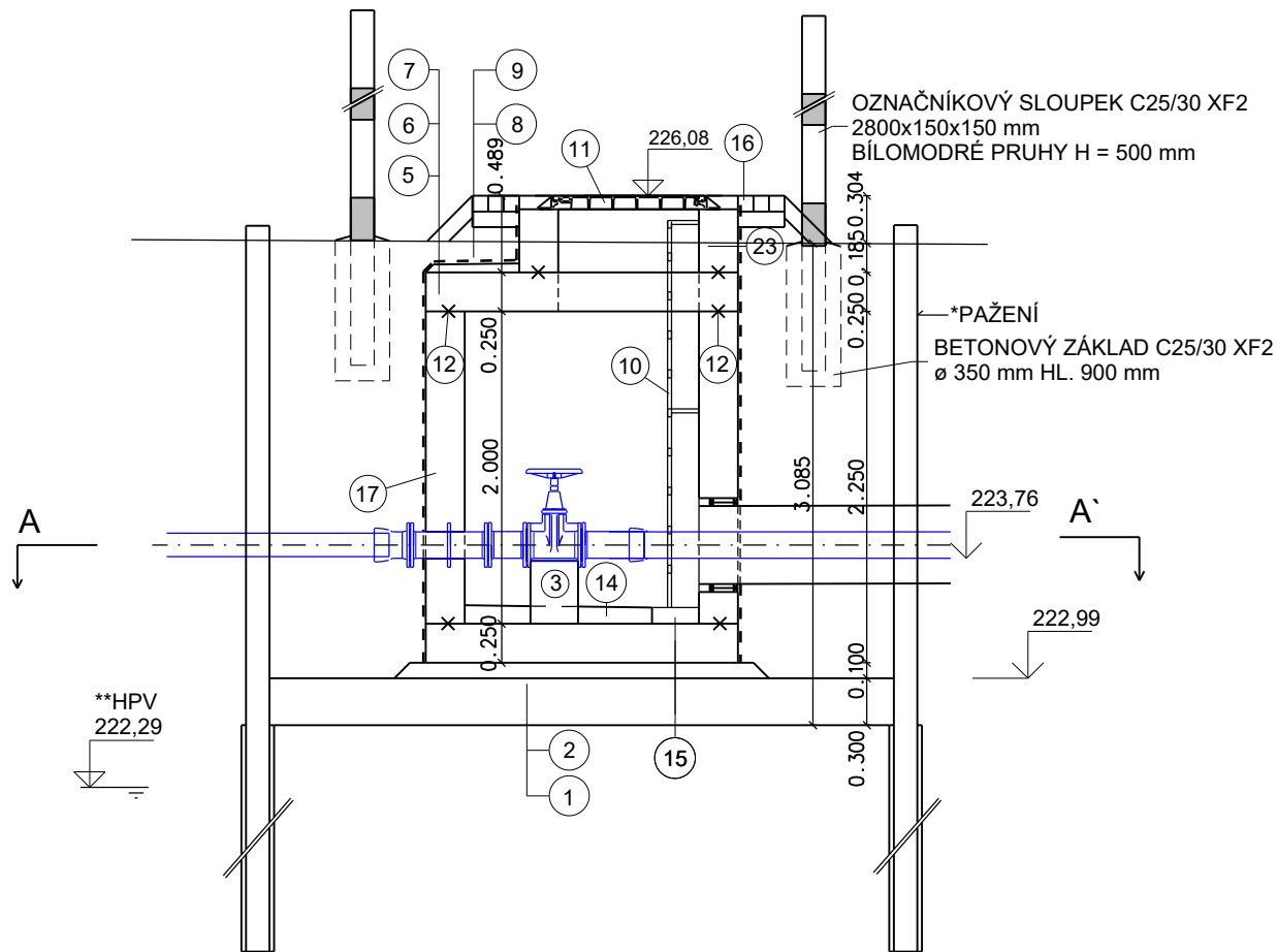
ŘEZ B - B´
