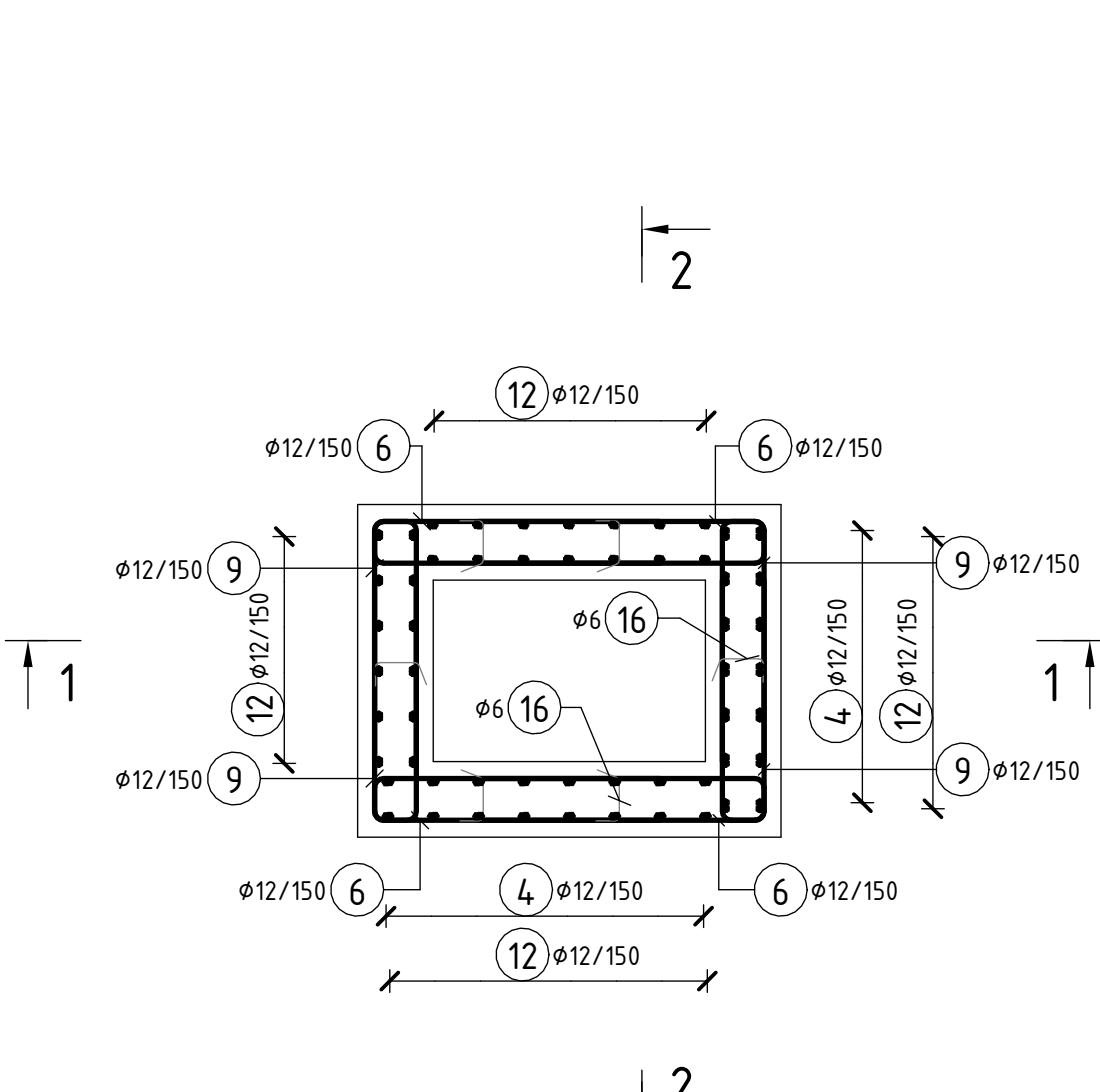
ŘEZ 4-4 1: 25
