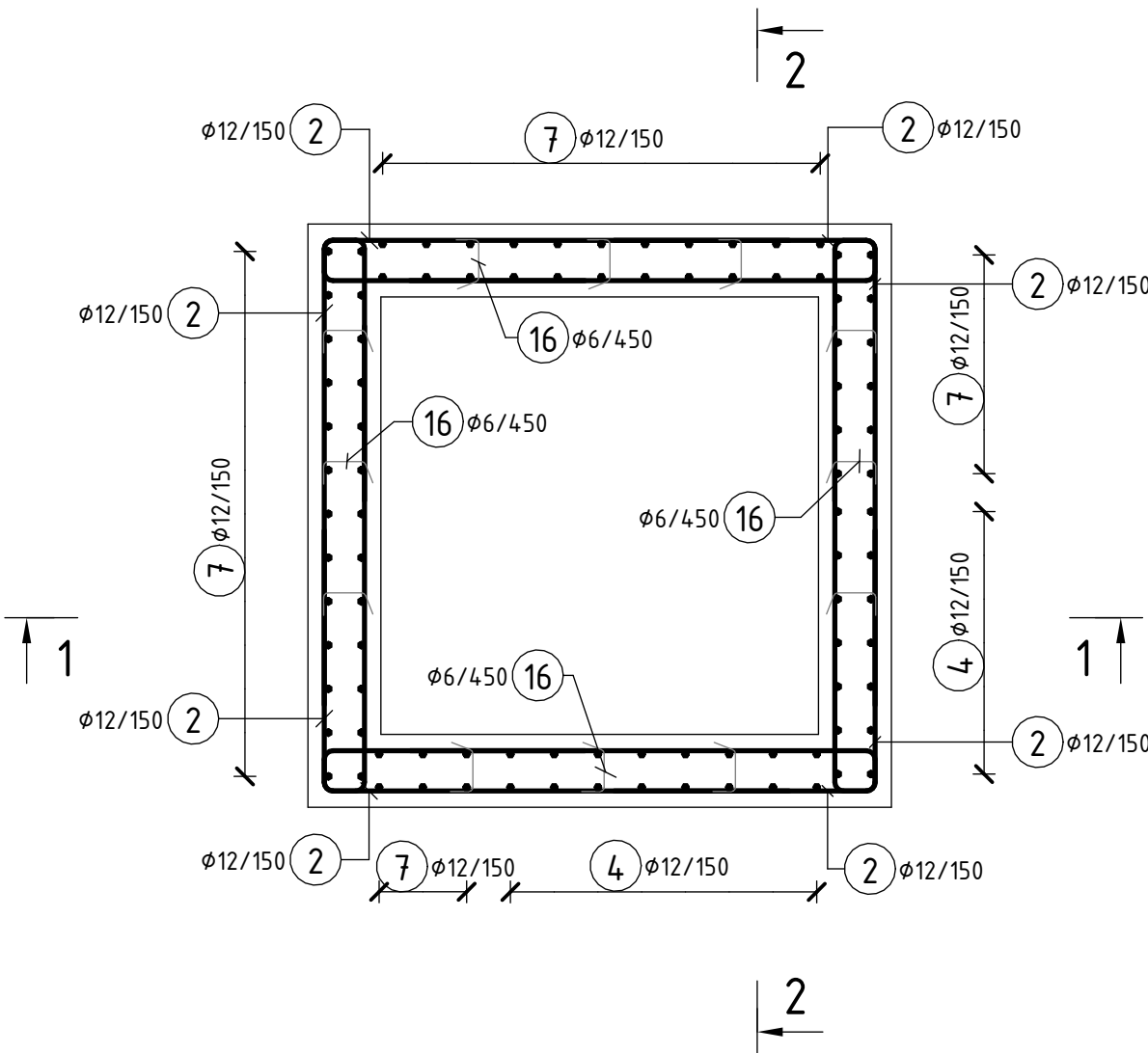
ŘEZ 3-3 1: 25
