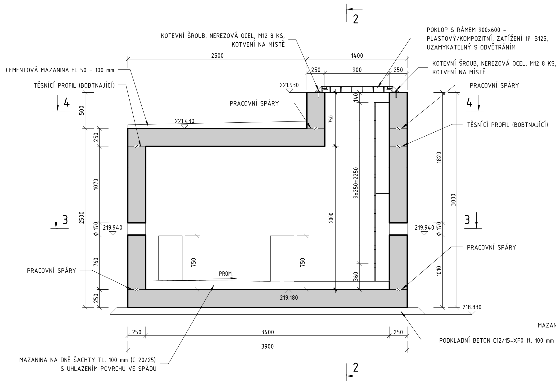
ŘEZ 1-1 1:25
