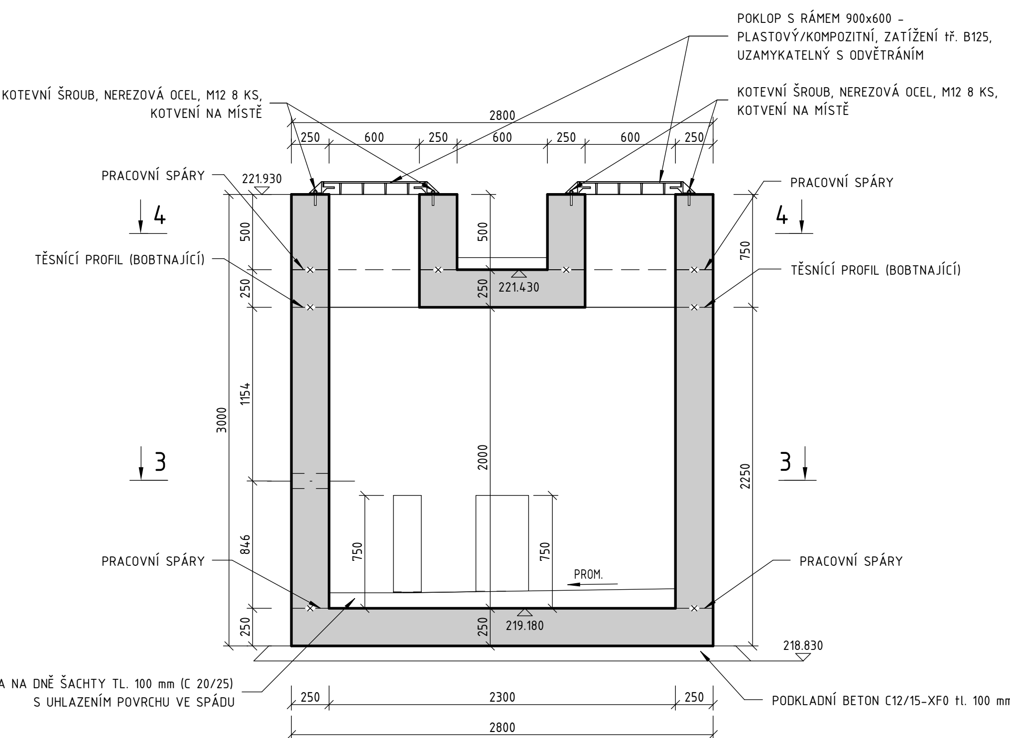
ŘEZ 2-2 1:25
