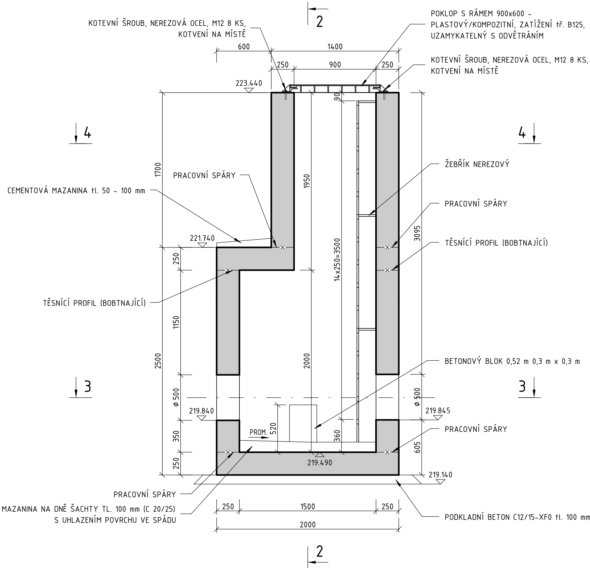
ŘEZ 1-1 1:25
