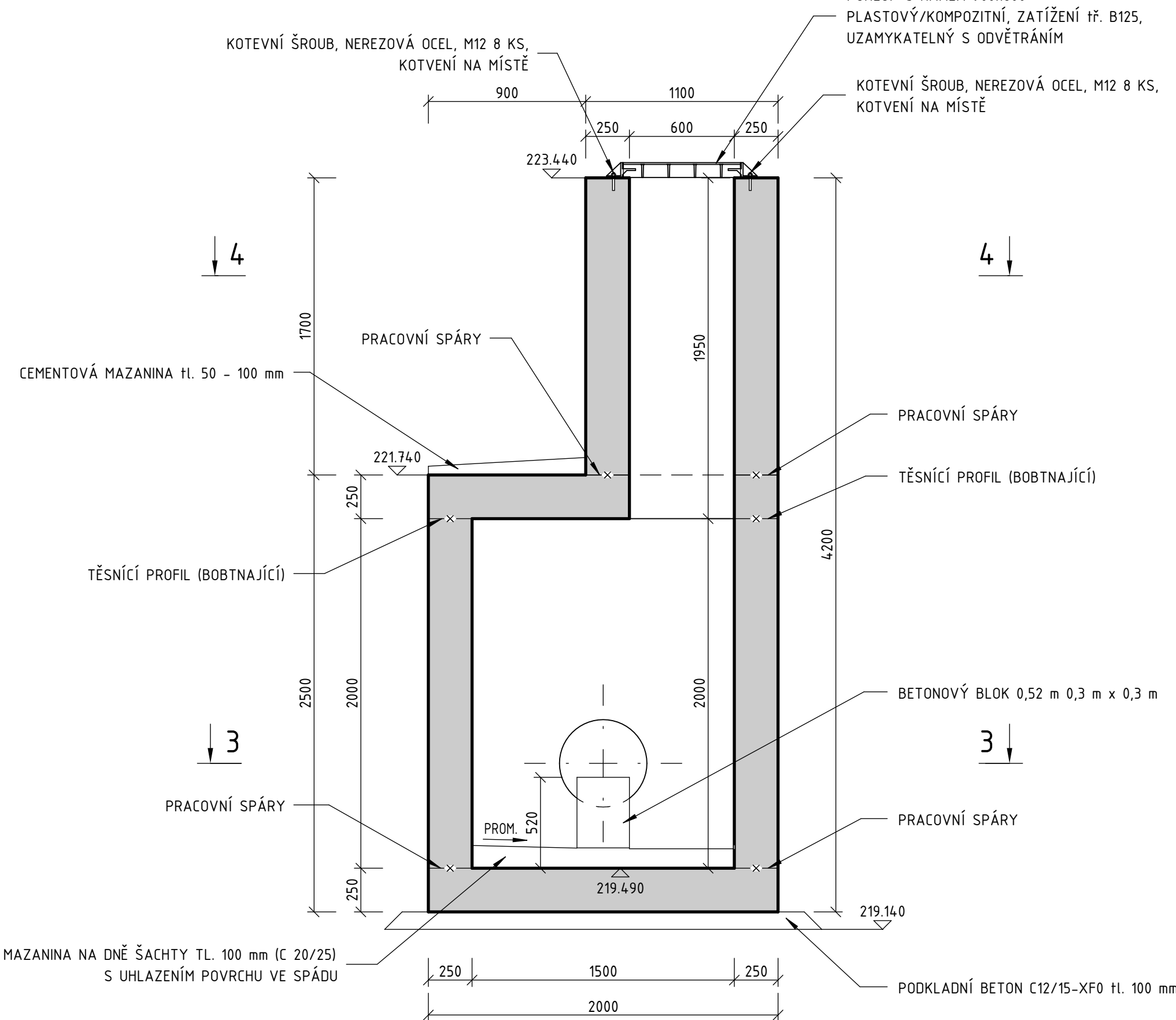
ŘEZ 2-2 1:25
