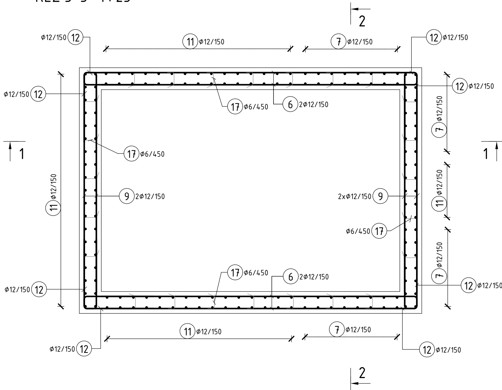
ŘEZ 3-3 1: 25
