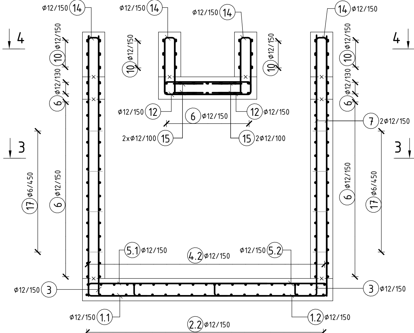
ŘEZ 2-2 1: 25
