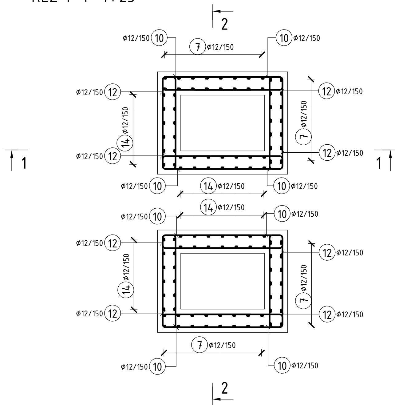
ŘEZ 4-4 1: 25
