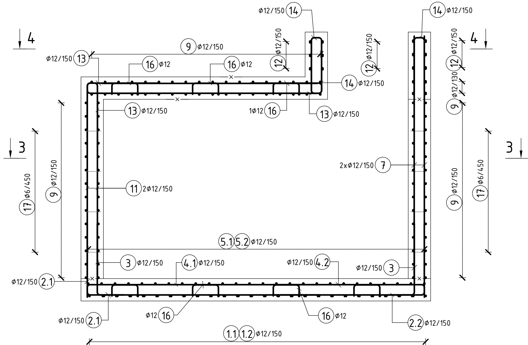
ŘEZ 1-1 1: 25
