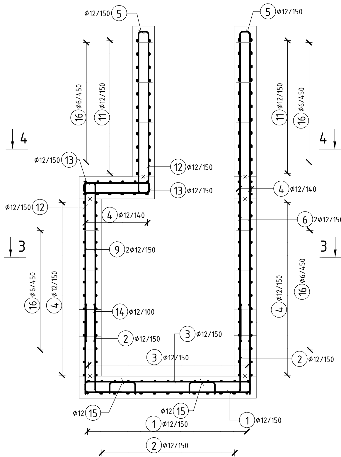
ŘEZ 1-1 1: 25
