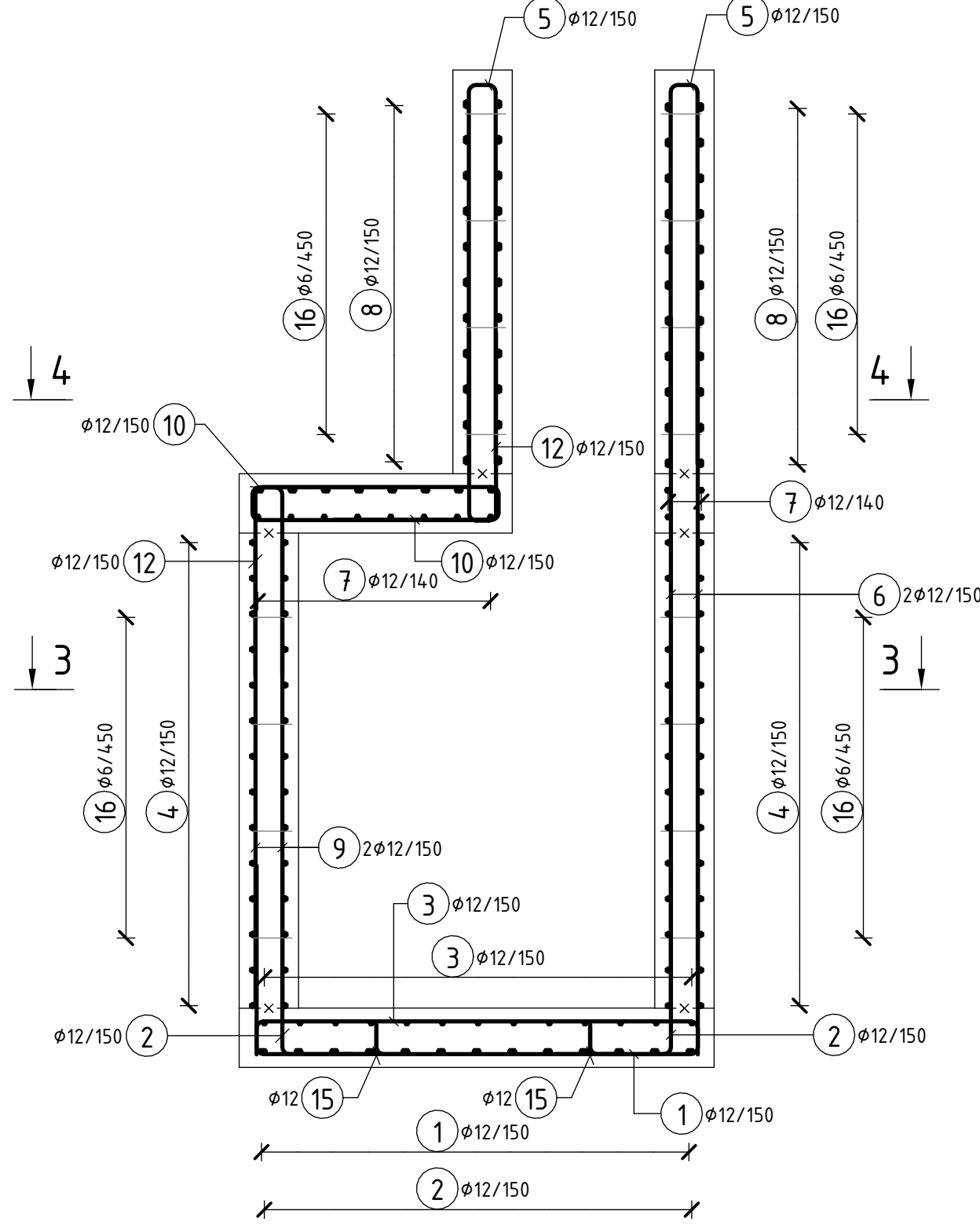
ŘEZ 2-2 1: 25
