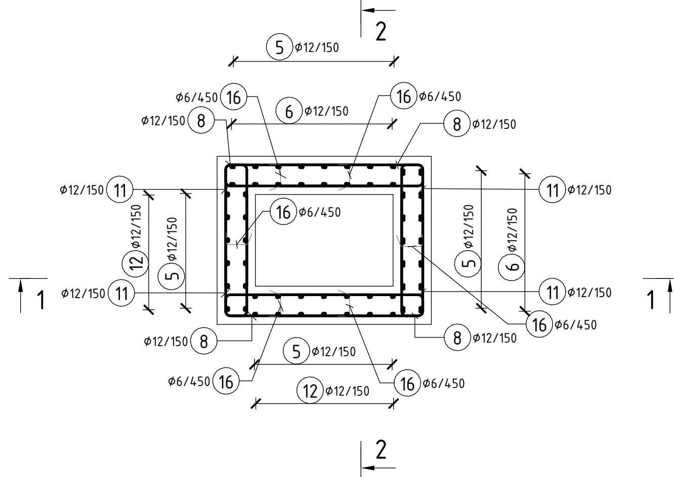
ŘEZ 4-4 1: 25
