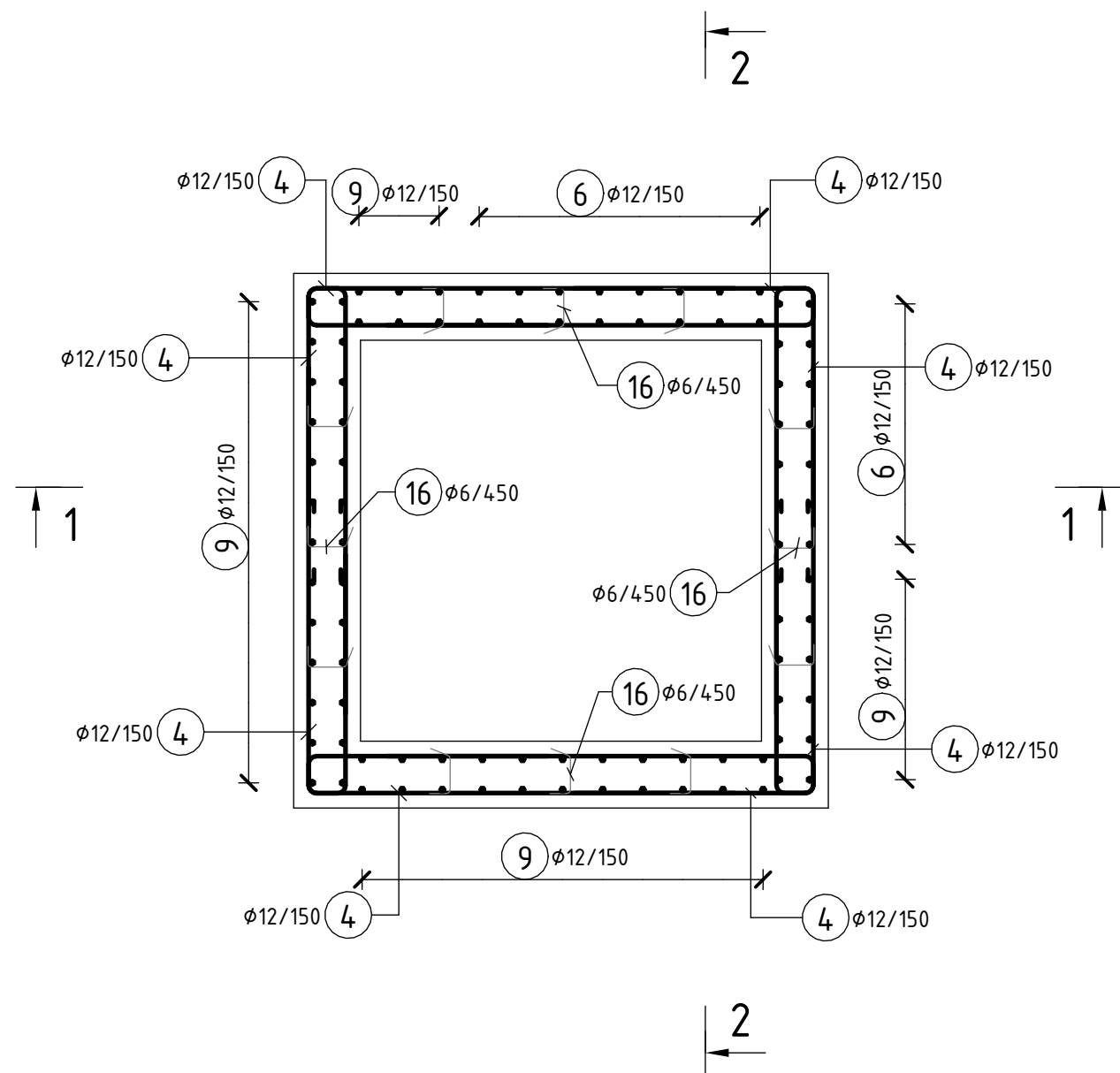
ŘEZ 3-3 1: 25
