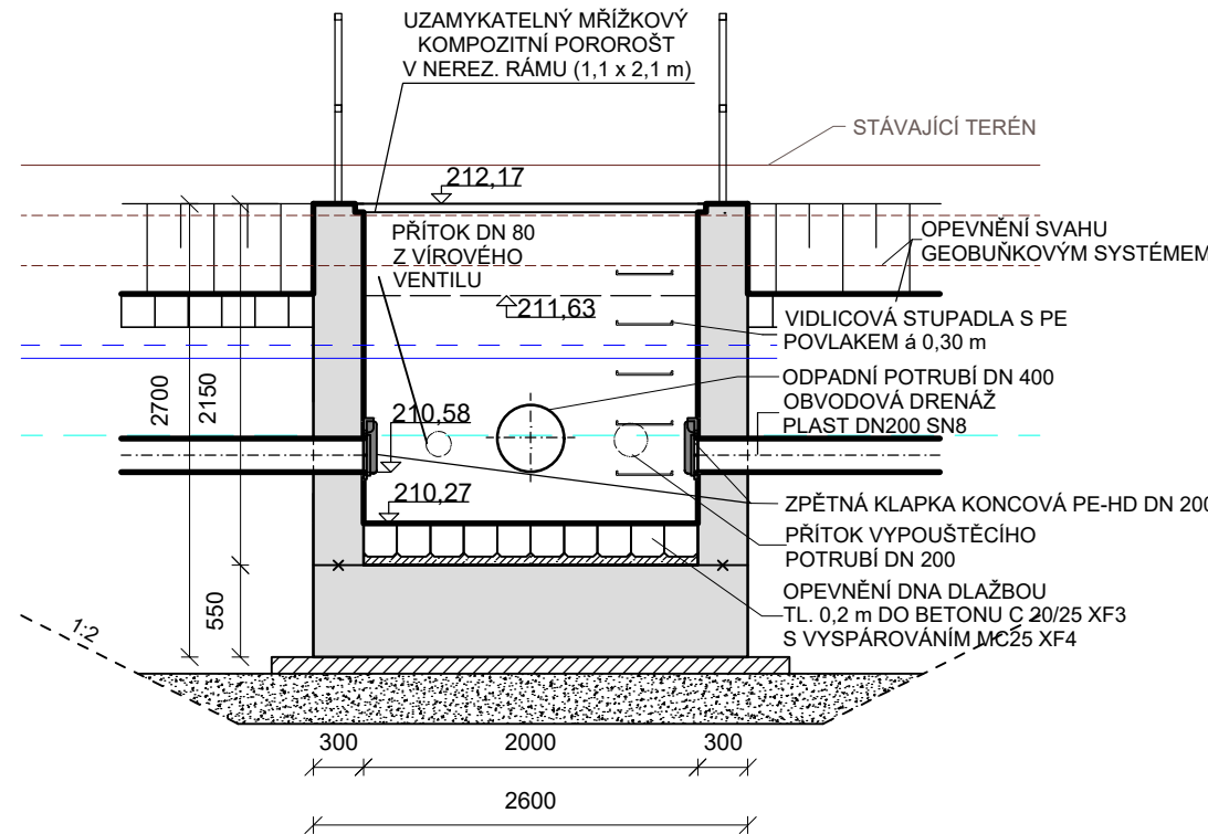
ŘEZ 1-1
