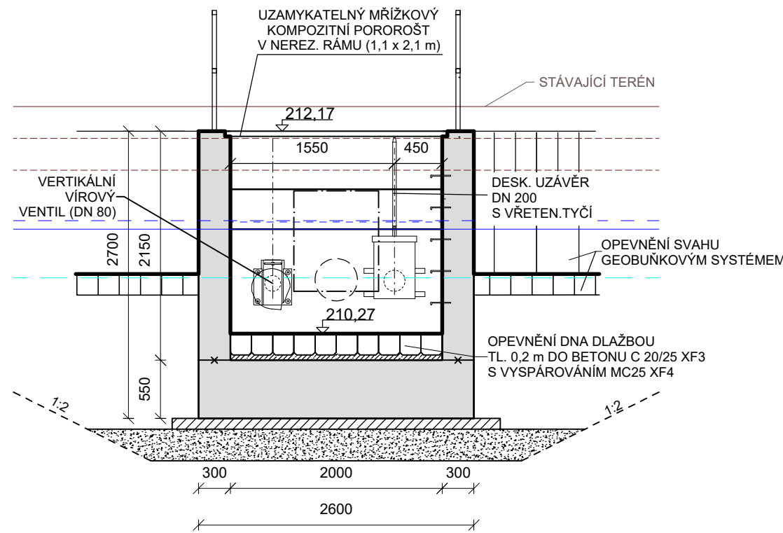
ŘEZ 1-1
