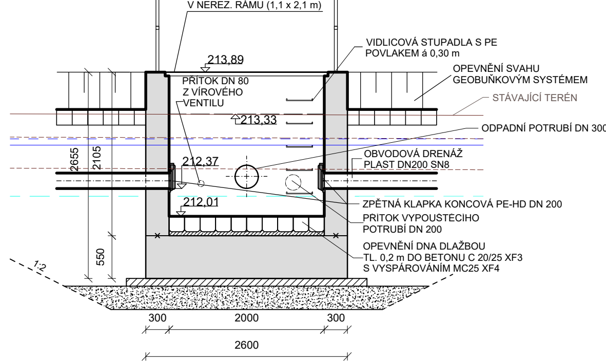
ŘEZ 1-1
