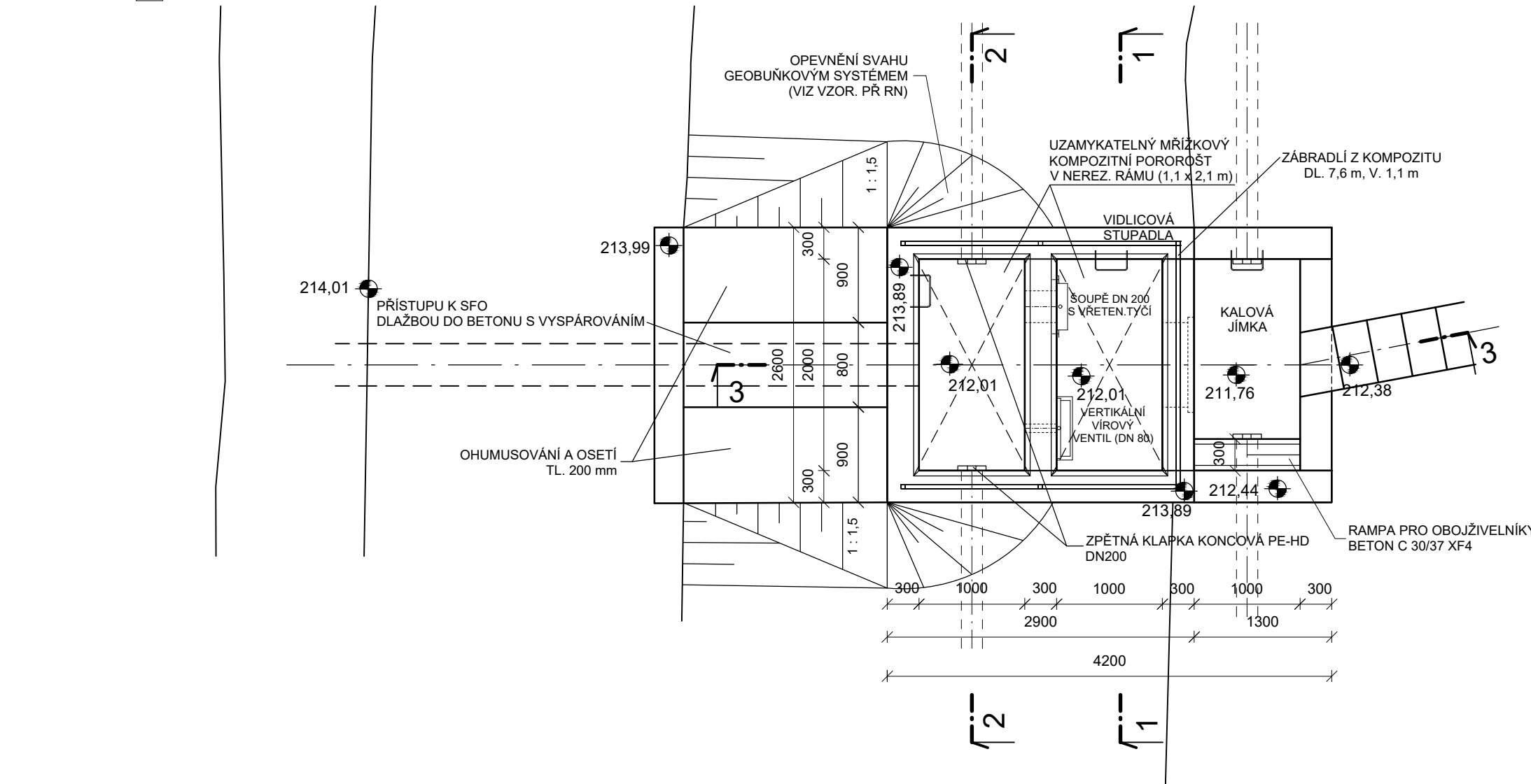
PŮDORYS
