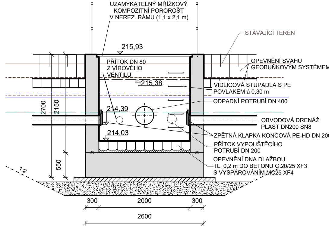
ŘEZ 2-2
