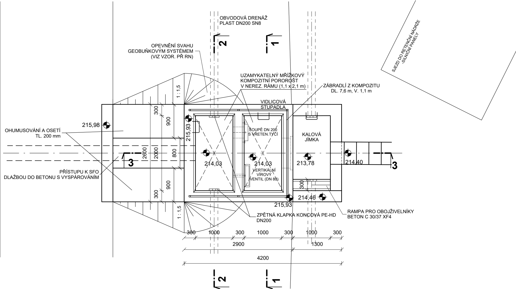
PŮDORYS
