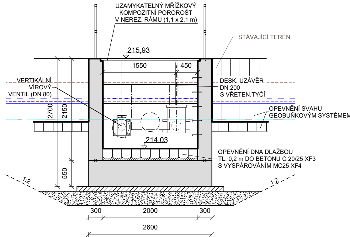
ŘEZ 1-1
