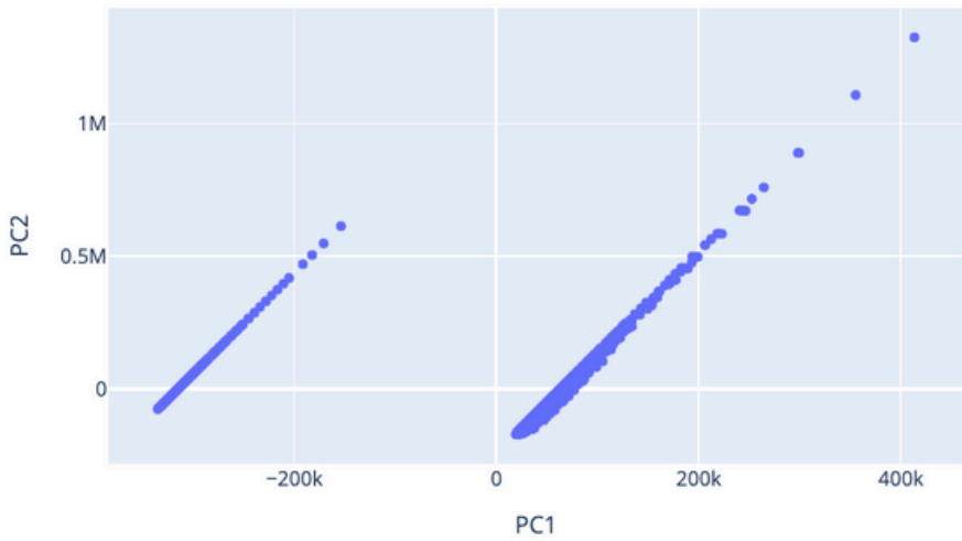
PCA 2D
