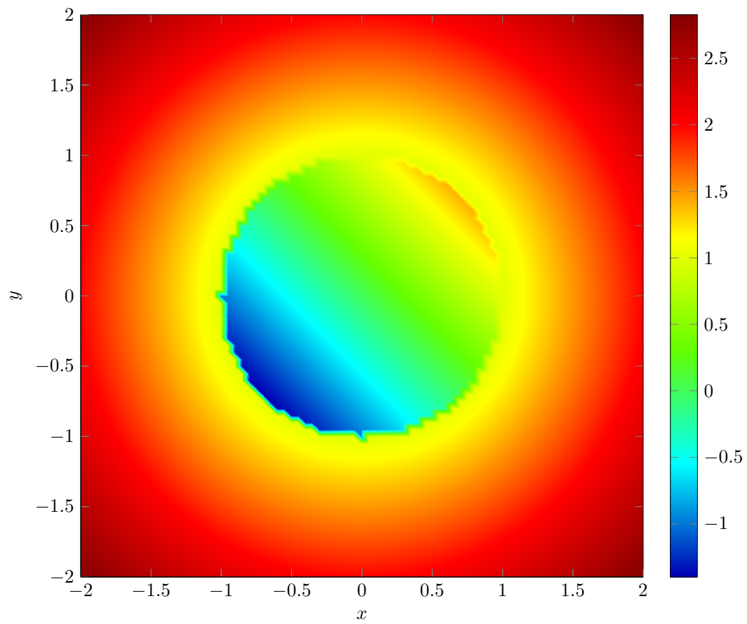
Кусочная функция двух переменных
