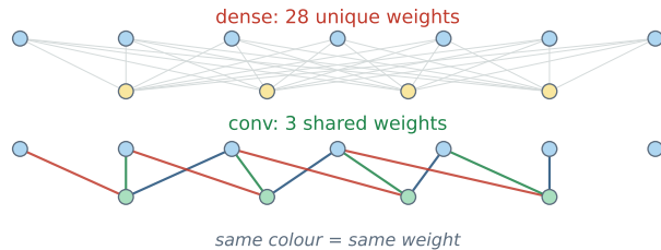
(a) parameter sharing
