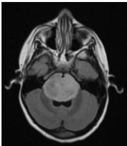
TEST Te-gl_160.jpg (557, 641)
