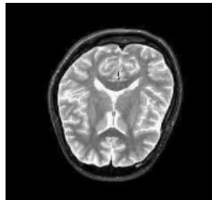
TEST Te-no_105.jpg (232, 217)
