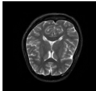
TRAIN Tr-no_294.jpg (232, 217)
