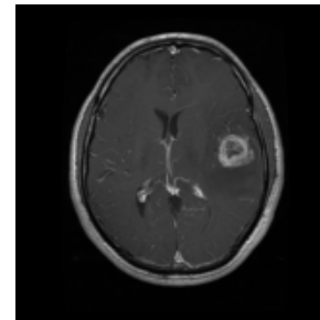
TEST Te-gl_214.jpg (512, 512)
