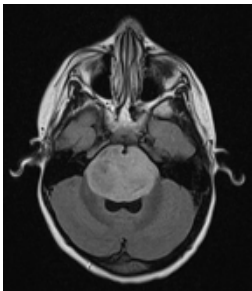
TRAIN Tr-me_1122.jpg (300, 345)
