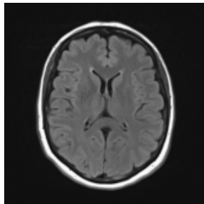
TEST Te-no_100.jpg (442, 442)
