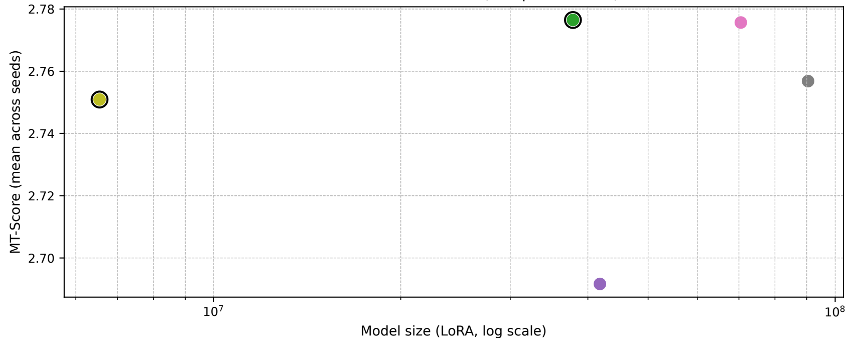
BPI20TPD - LLM LoRA Pareto (best per backbone)
