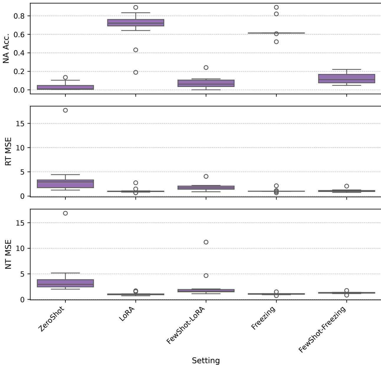
Backbone: llama32-1b
