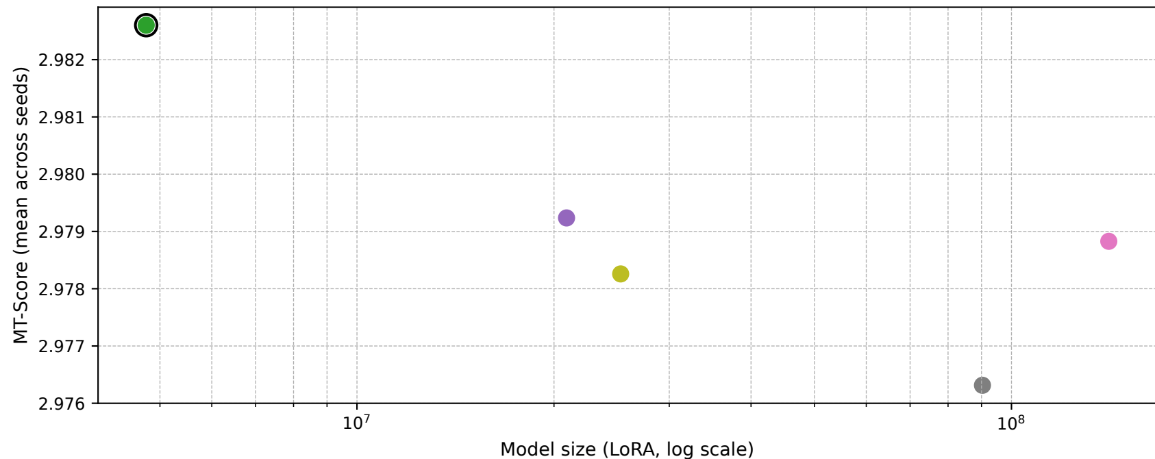
BPI20RfP - LLM LoRA Pareto (best per backbone)
