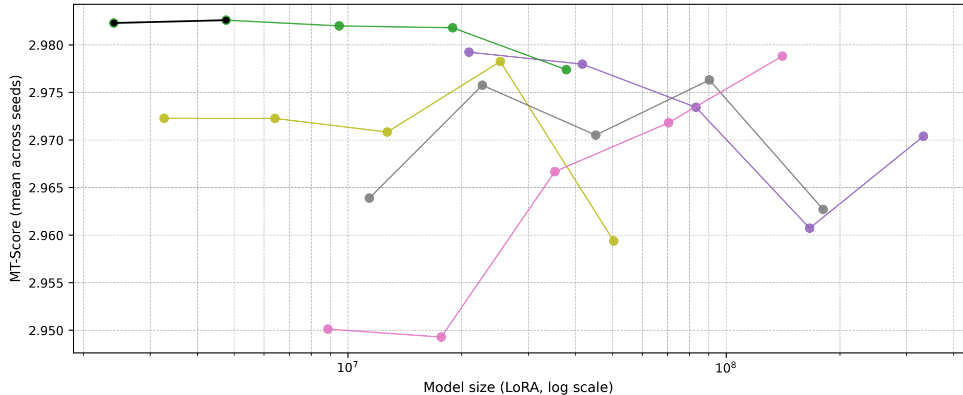
BPI20RfP - LLM LoRA sweeps (Pareto front)
