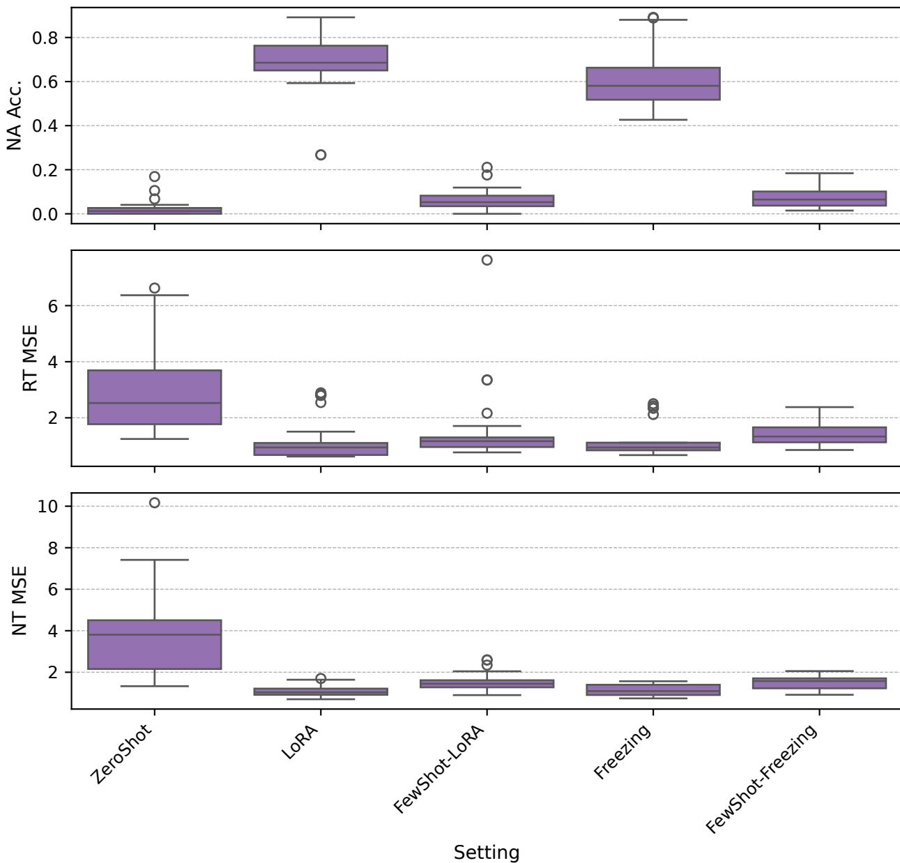
Backbone: gptneo-1b3
