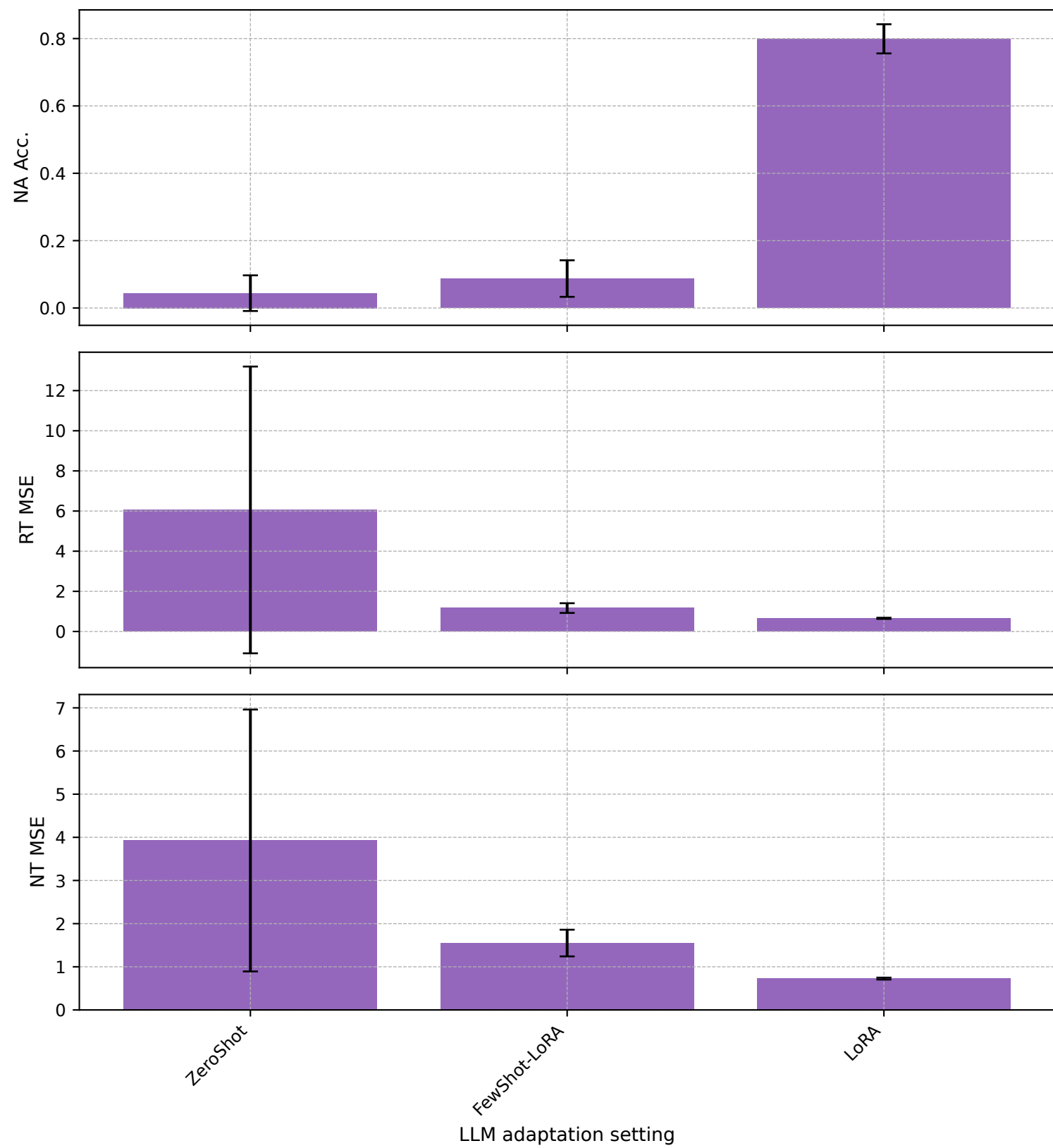
BPI17 - llama32-1b
