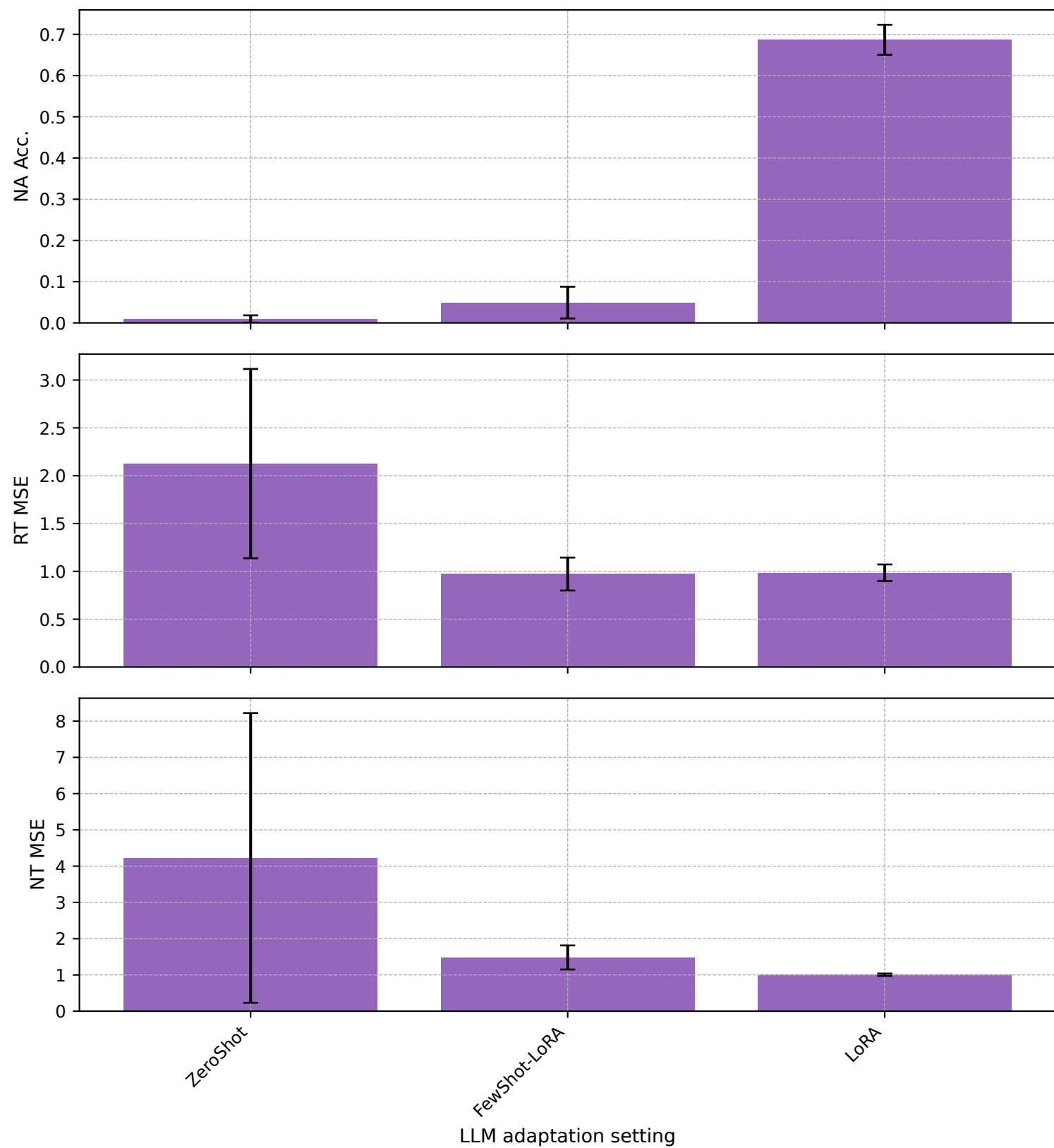
BPI20TravelPermitData - gptneo-1b3
