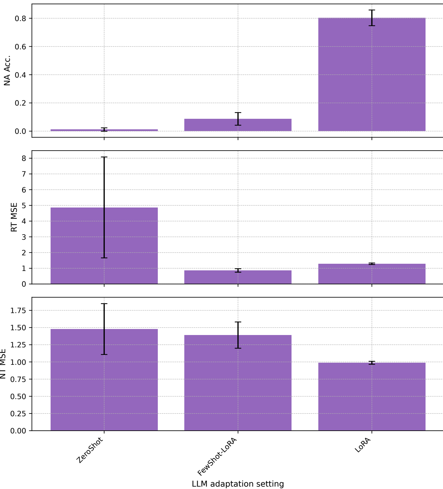
BPI17 - gpt2
