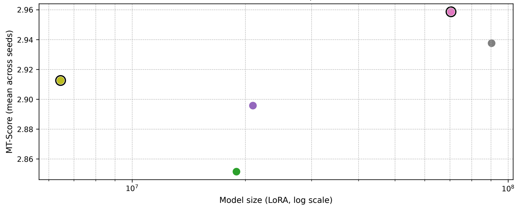
BPI17 - LLM LoRA Pareto (best per backbone)
