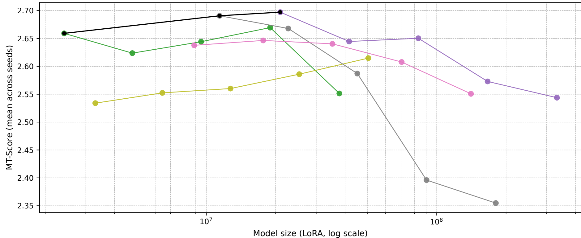
BPI12 - LLM LoRA sweeps (Pareto front)
