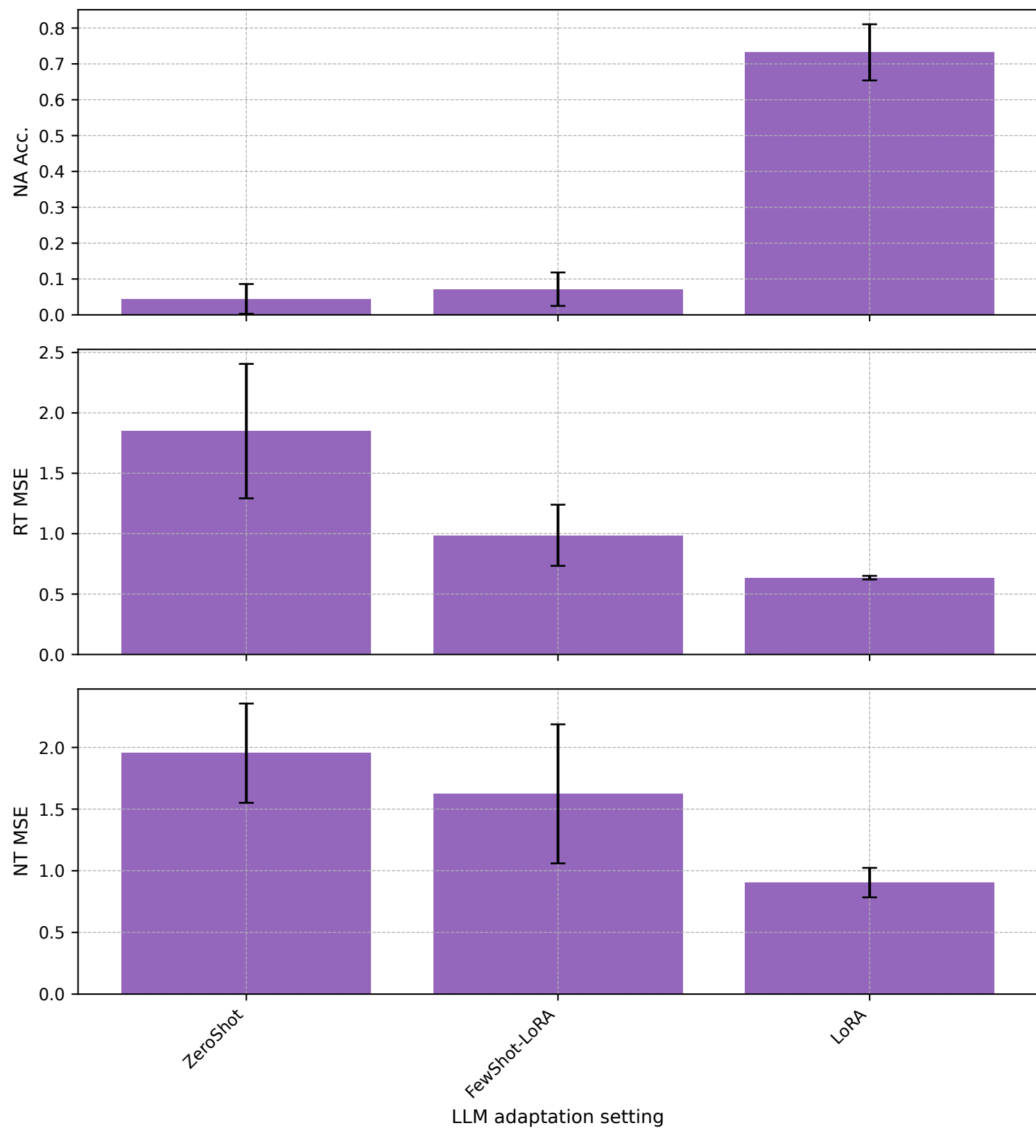
BPI17 - gptneo-1b3
