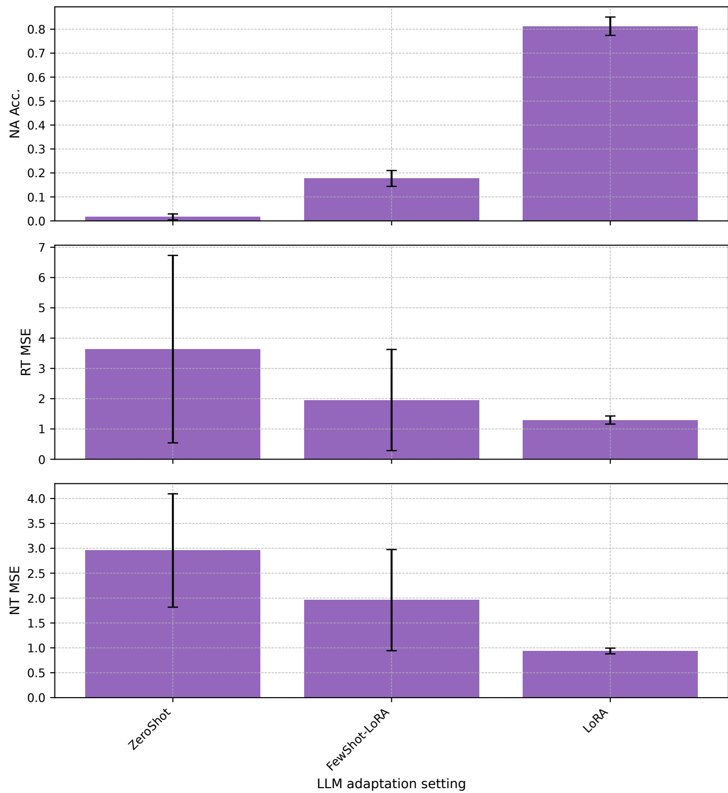
BPI17 - gemma-2-2b
