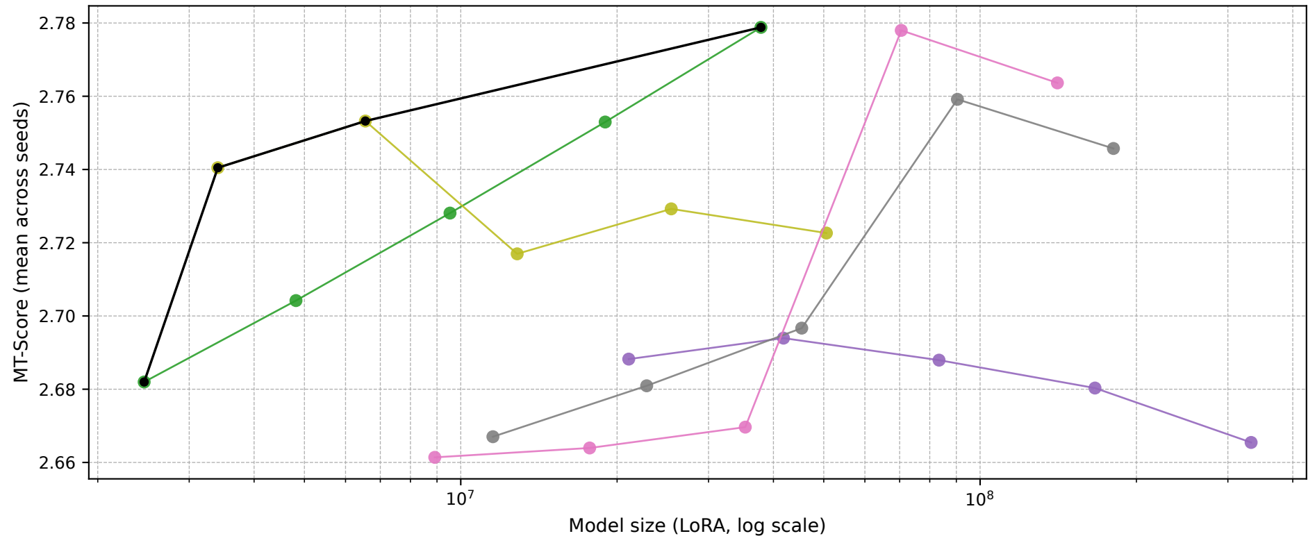
BPI20TPD - LLM LoRA sweeps (Pareto front)
