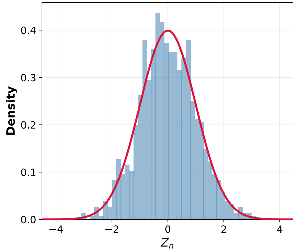
D1 Linear, n = 100
