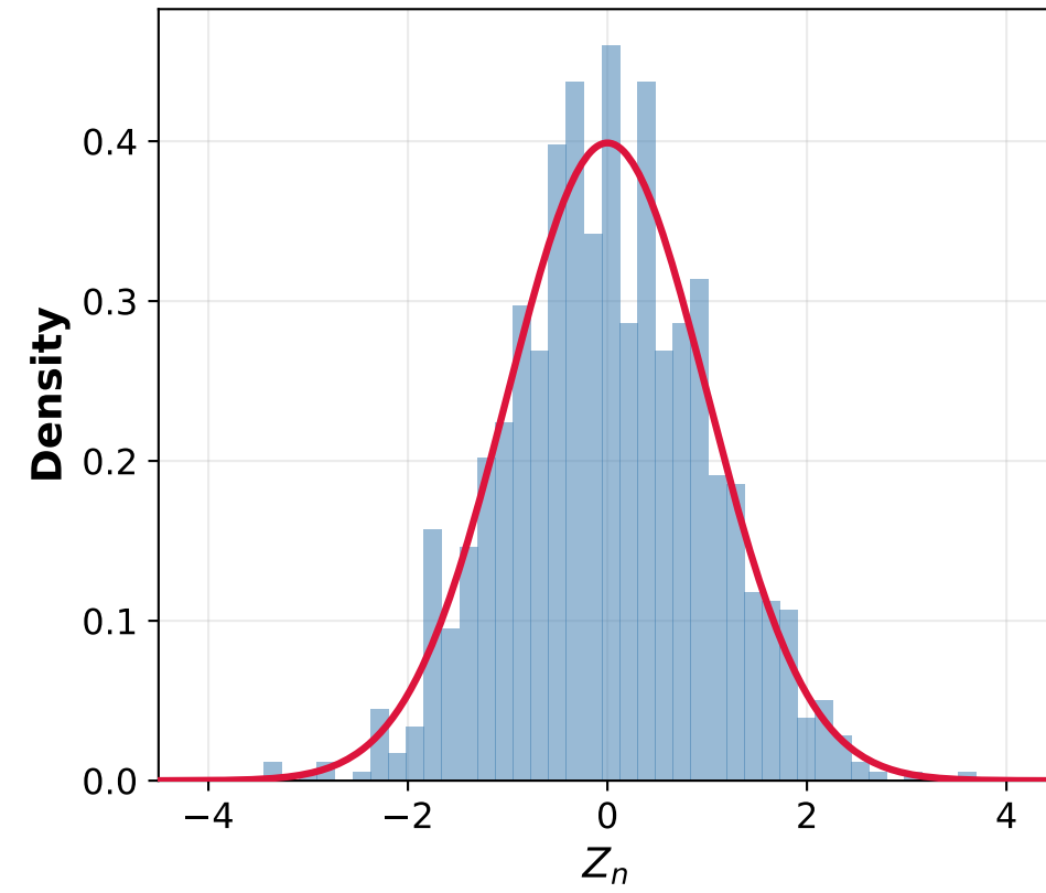
D1 Linear, n = 500
