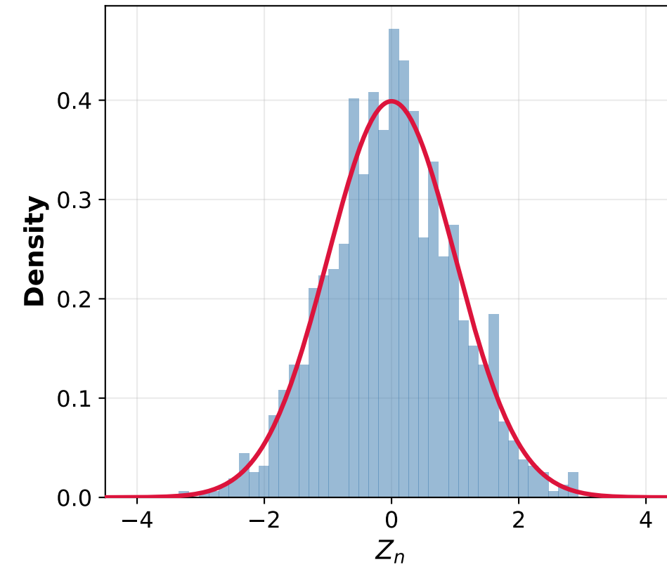
D1 Linear, n = 1000
