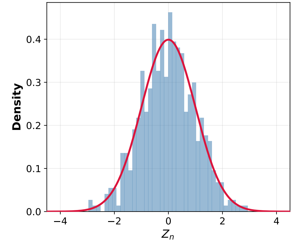
D1 Linear, n = 5000
