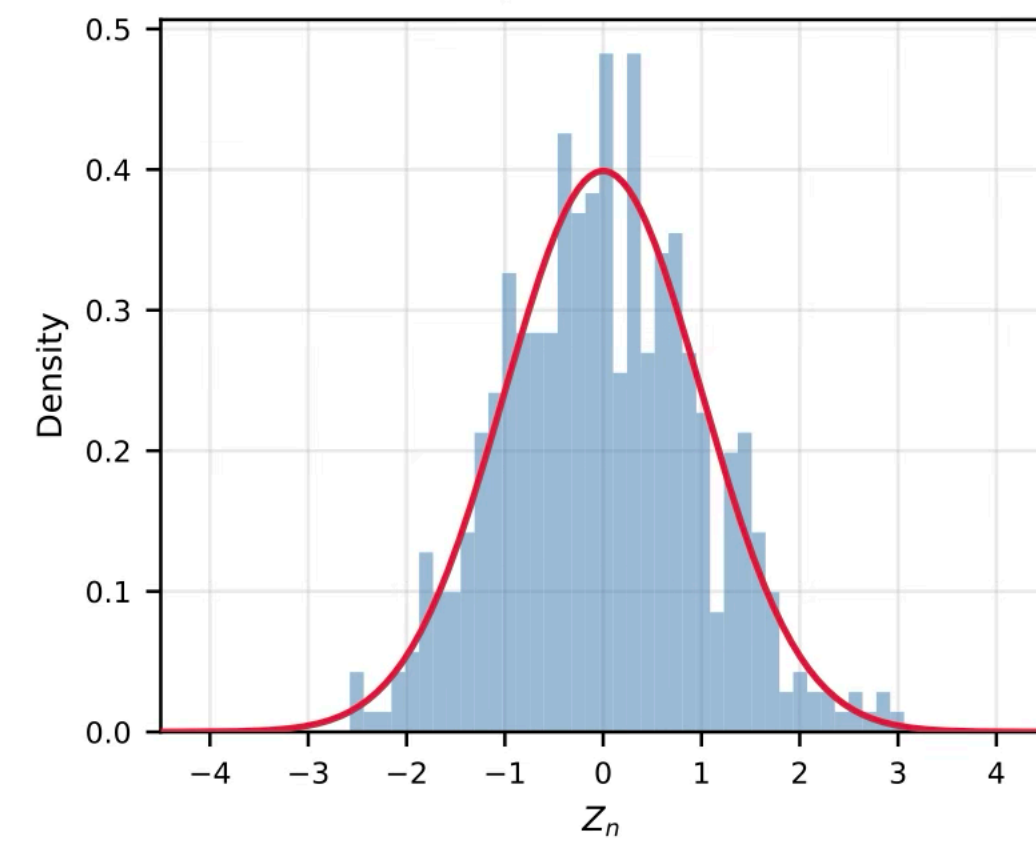
D1 Linear, n = 5000
