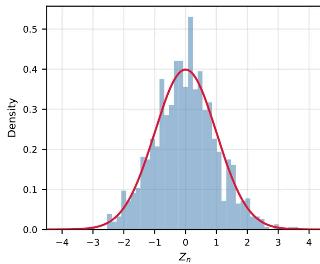
D1 Linear, n = 1000
