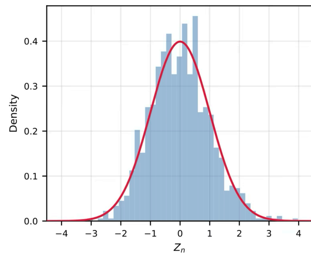
D1 Linear, n = 100
