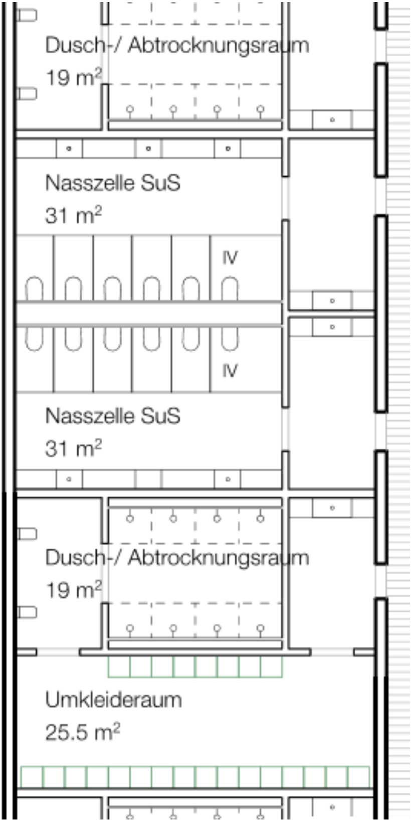
Nasszellen / Garderoben / Du
