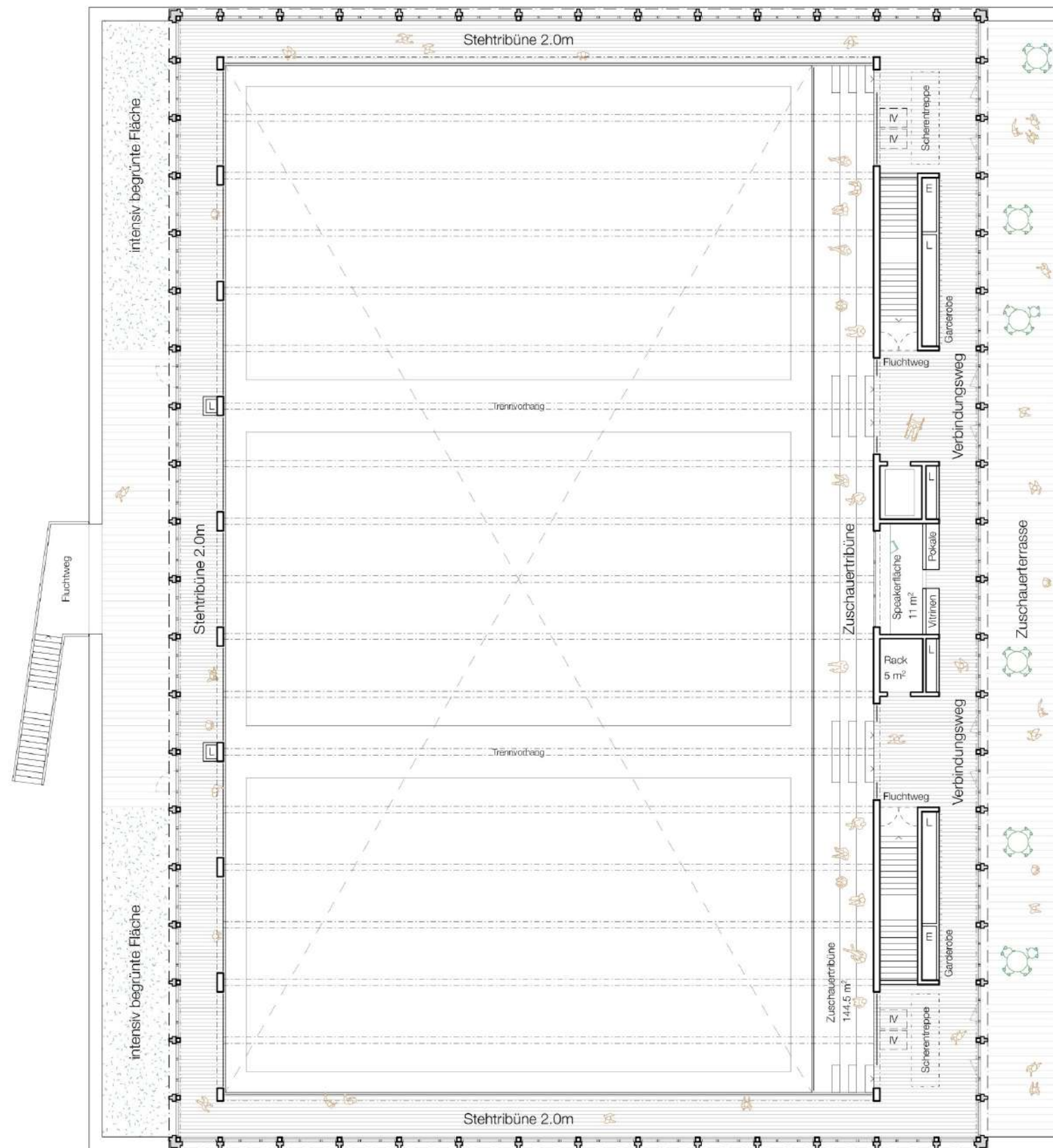
Obergeschoss
