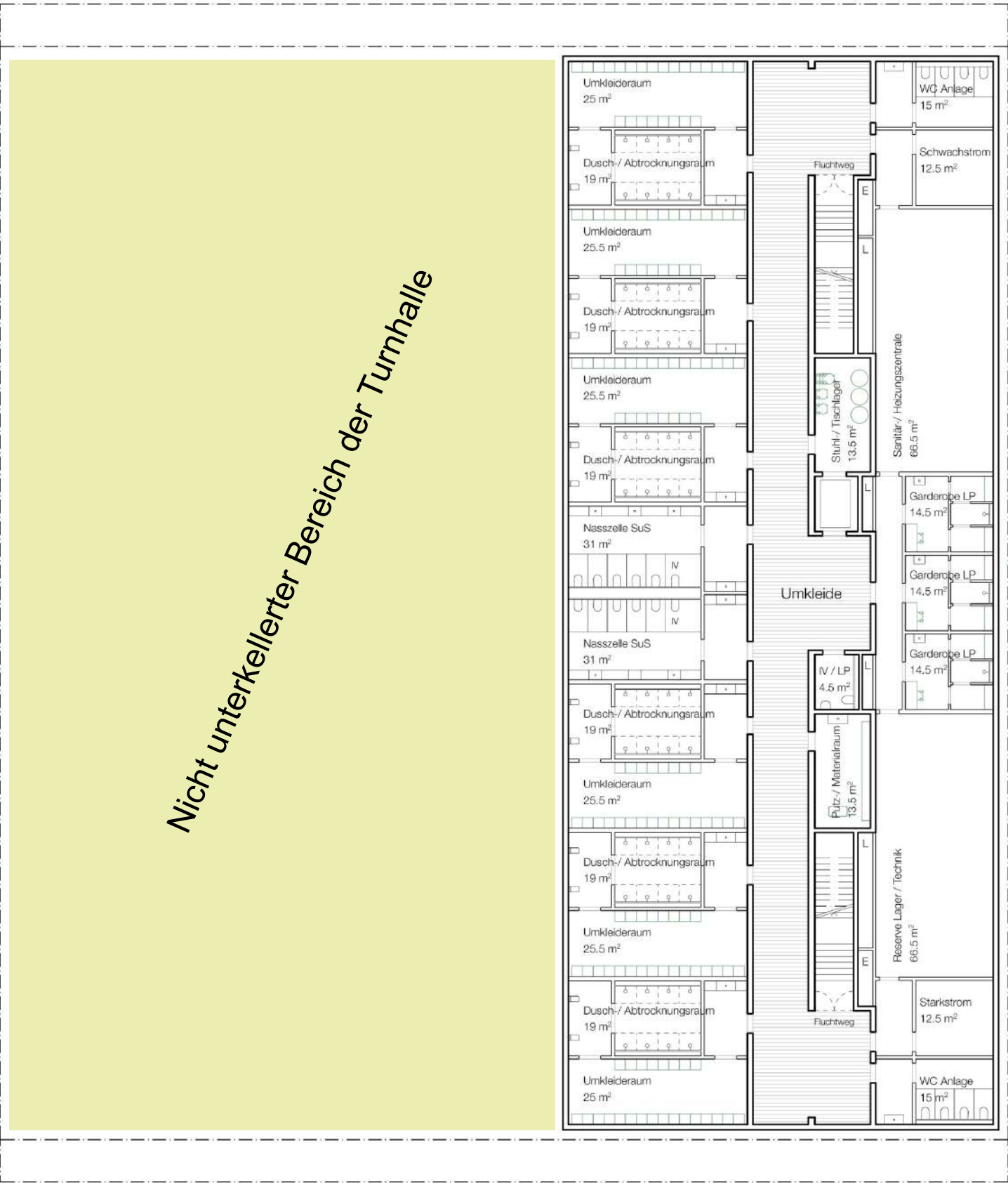
Untergeschoss
