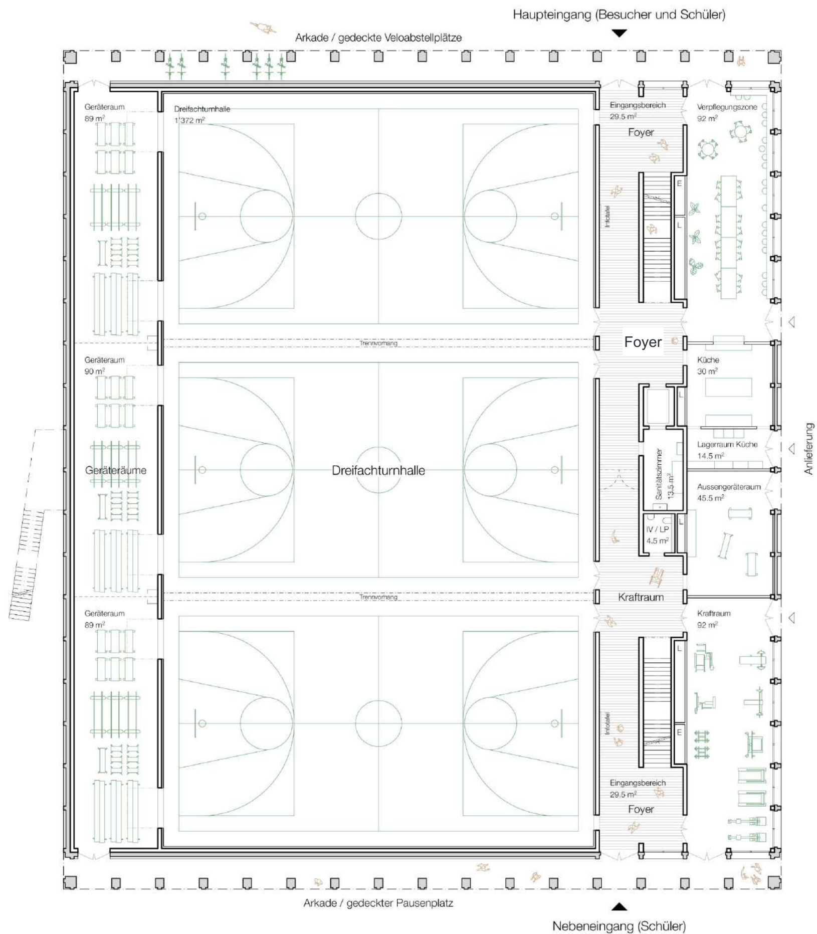
Erdgeschoss
