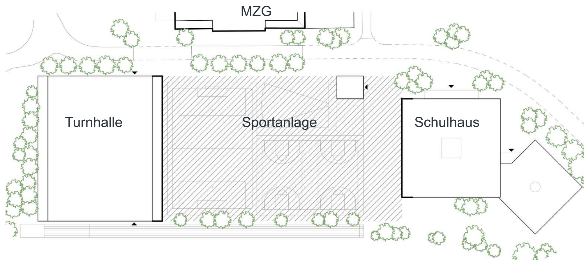
Sportanlage als gemeinschaftliche Mitte
