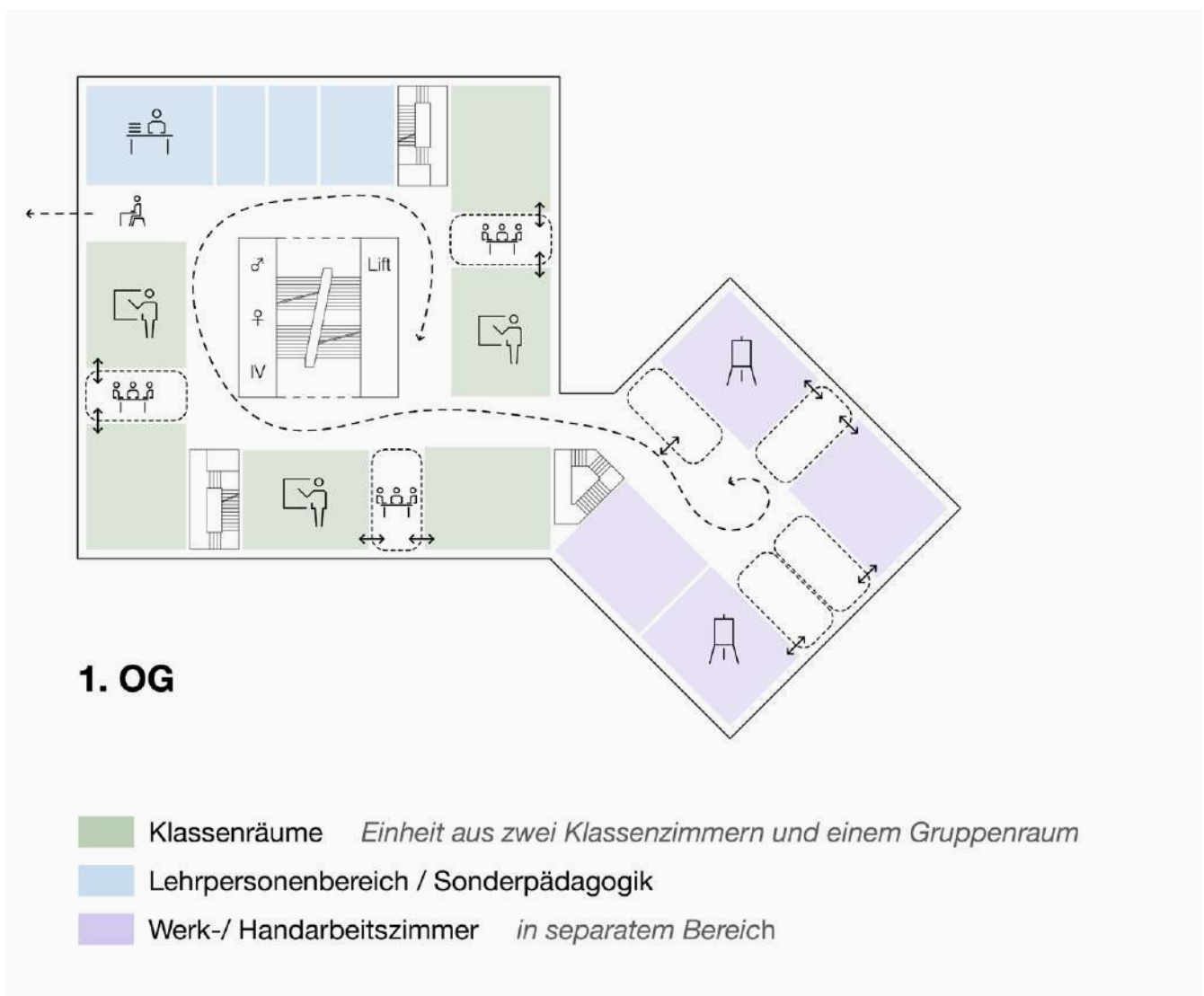
Abb. 9: 1. Obergeschoss Raumteilung
