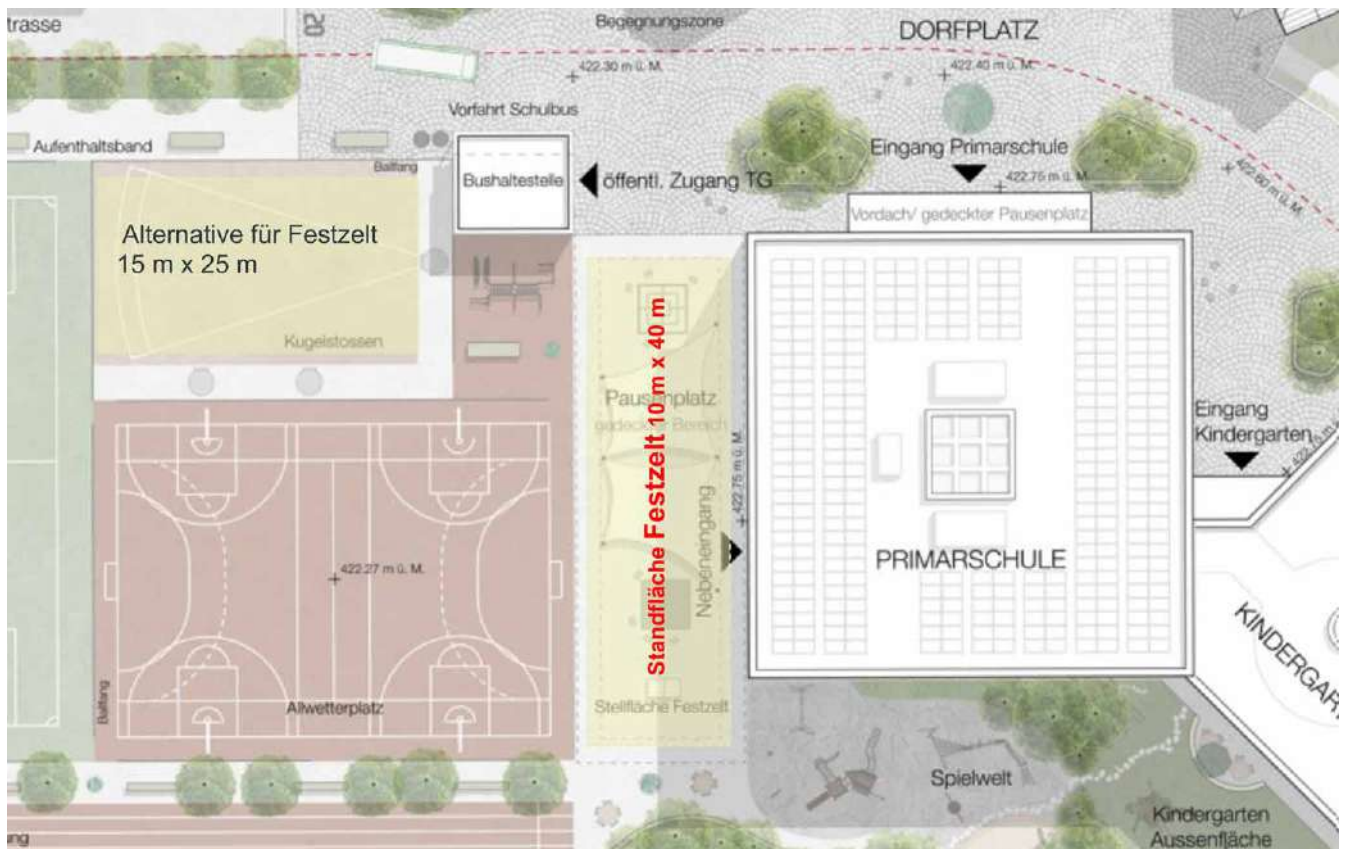
Abb. 33: Festzeltstandflächen
