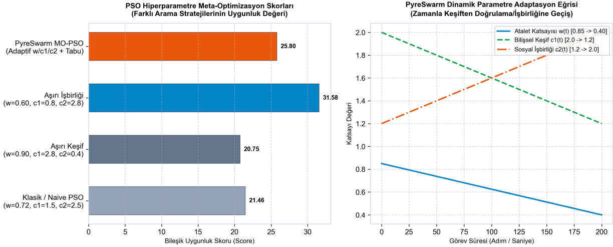
Şekil 2: PSO Hiperparametre Meta-Optimizasyon Skorları ve Dinamik Parametre Adaptasyon Eğrileri
