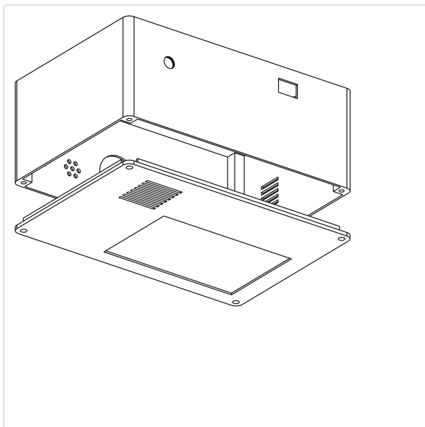
Figure 7 — Modèle 3D paramétrique (base et couvercle, vue éclatée) généré par fablab/boitier.py , importé dans Fusion 360 pour la finition.
