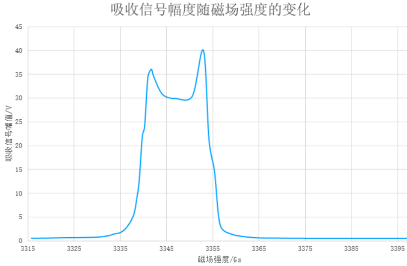
图 14: 直接法测量吸收信号
