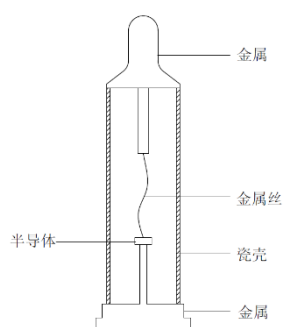
图 8 晶体检波器结构
