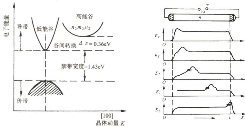
图 5 砷化镓的能带结构 图 6 耿式管中畴的形成、传播和消失过程
