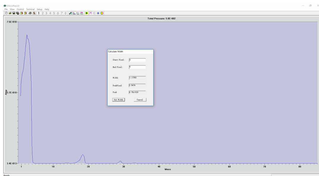
图 21: 真空度为 8.4 \times 10^{-3} Pa 改变分辨率为 60，发射电压为 40 下的扫描结果
