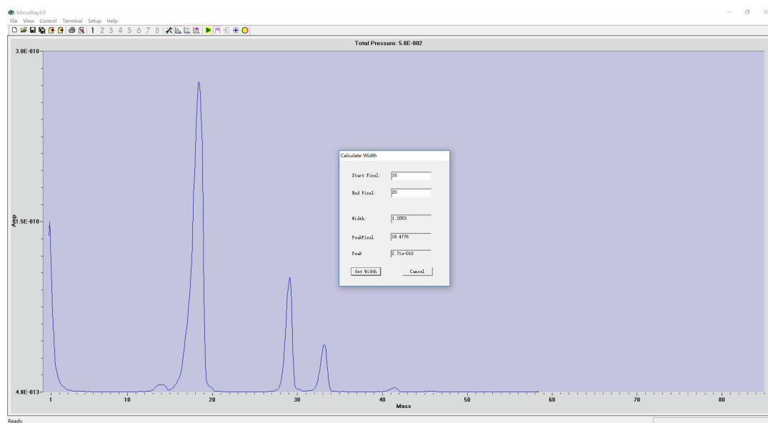
图 28: 真空度为 6.8 \times 10^{-3} Pa 改变发射系数为 0.2, 发射电压为 40 下的扫描结果
