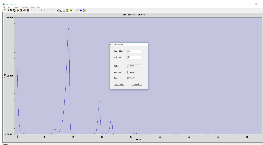
图 30: 真空度为 7.6 \times 10^{-3} Pa 改变发射系数为 0.2, 发射电压为 60 下的扫描结果
