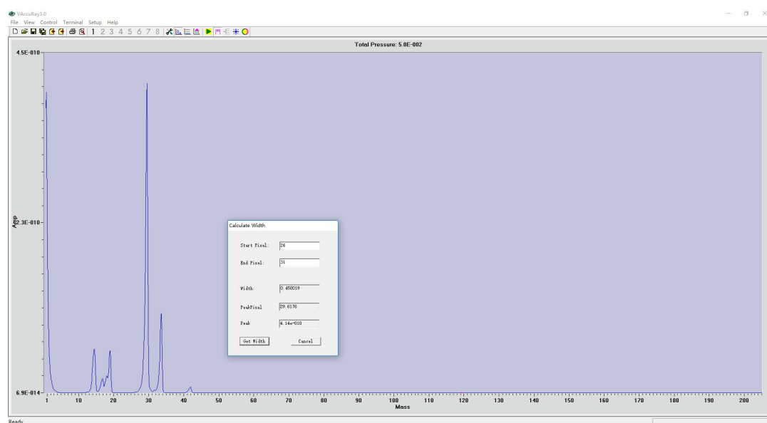
图 10: 真空度为 1 \times 10^{-2} Pa 改变分辨率为 30 下的扫描结果
