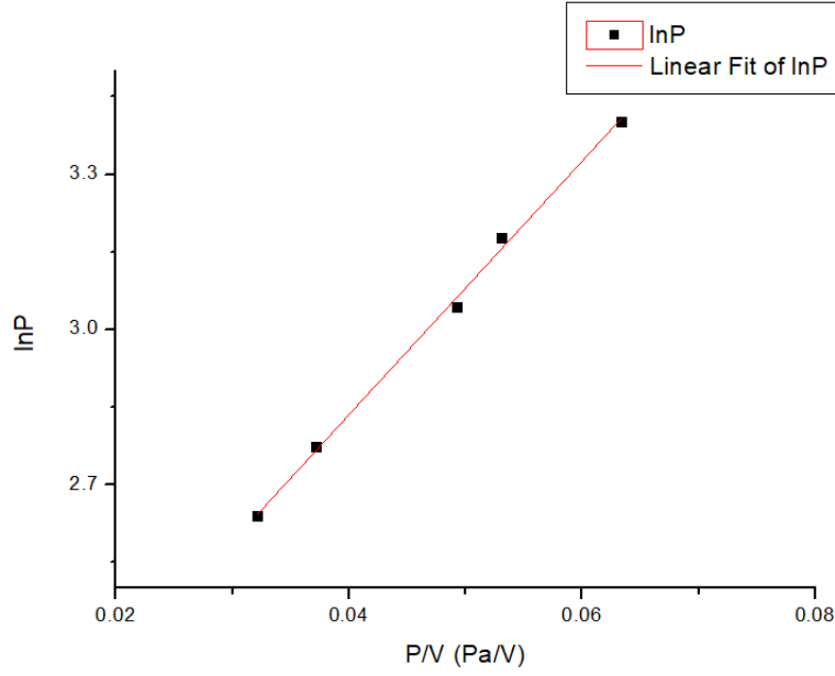
图 8: 极板间距为 4 cm 时的 p/V - \ln P 回归直线
