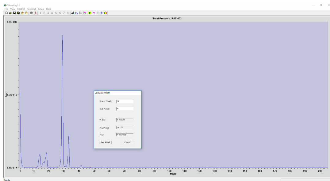
图 11: 真空度为 0.96 \times 10^{-2} Pa 改变分辨率为 60, 发射系数为 0.1 下的扫描结果
