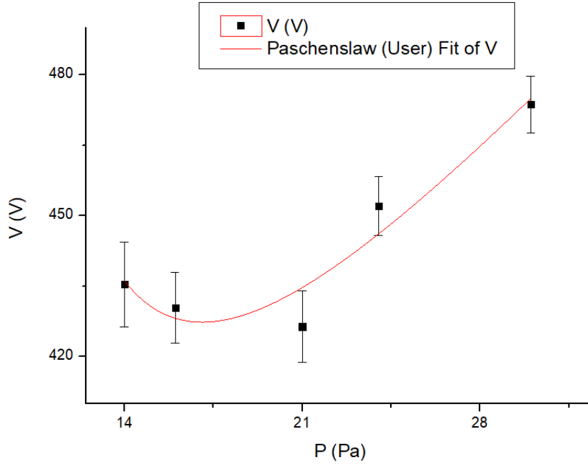
图 6: 极板间距为 4 cm 时的 p - V 曲线
