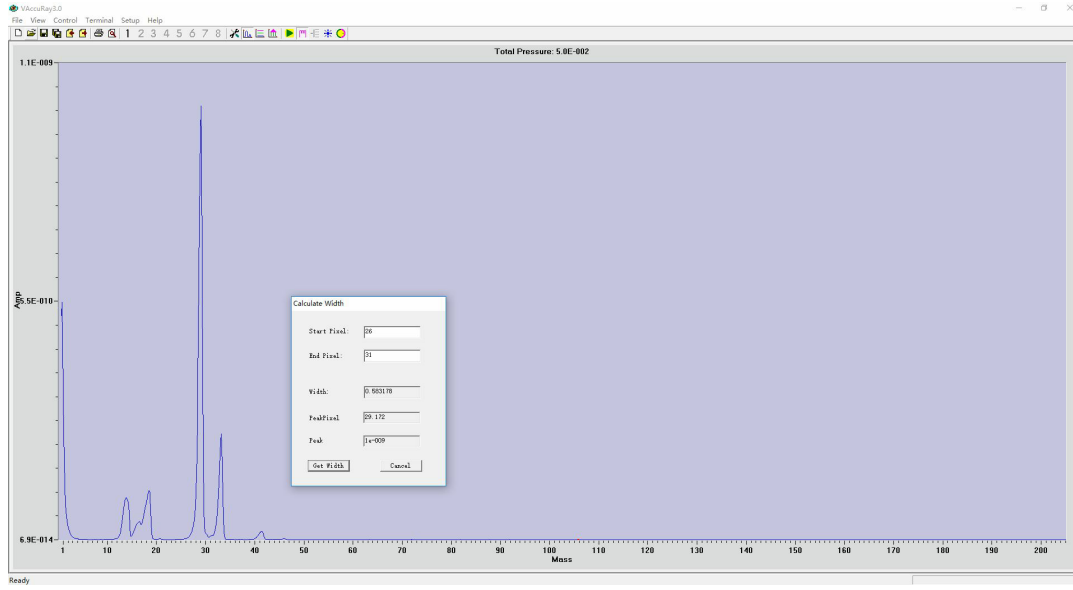
图 19: 真空度为 0.96 \times 10^{-2} Pa 改变分辨率为 60 下的扫描结果
