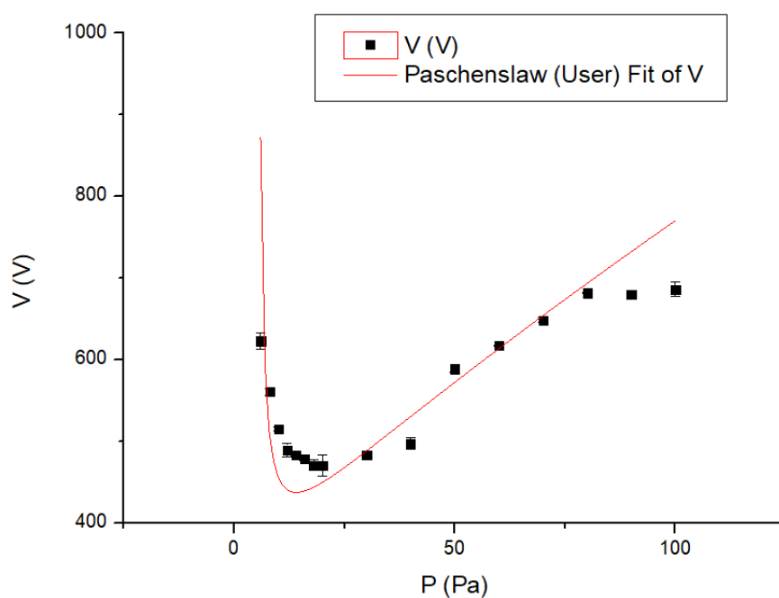
图 5: 极板间距为 5 cm 时的 p - V 曲线
