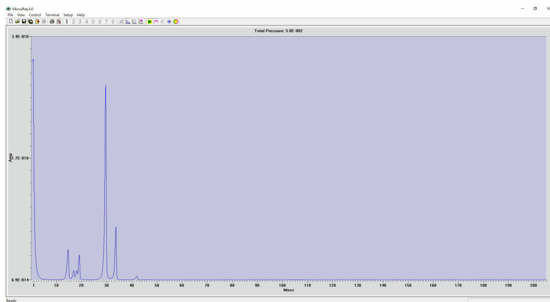
图 15: 真空度为 0.98 \times 10^{-2} Pa 改变分辨率为 20 下的扫描结果
