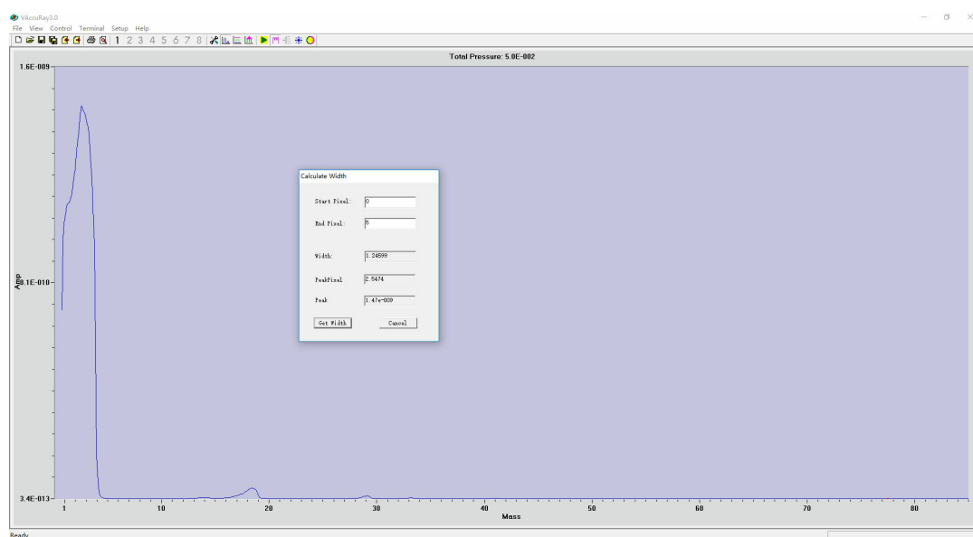
图 21: 真空度为 8.4 \times 10^{-3} Pa 改变分辨率为 60，发射电压为 80 下的扫描结果
