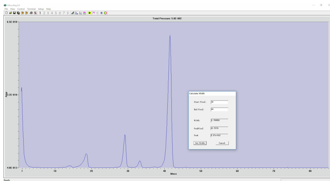
图 22: 真空度为 6.8 \times 10^{-3} Pa 改变发射系数为 0.2, 发射电压为 40 下的扫描结果
