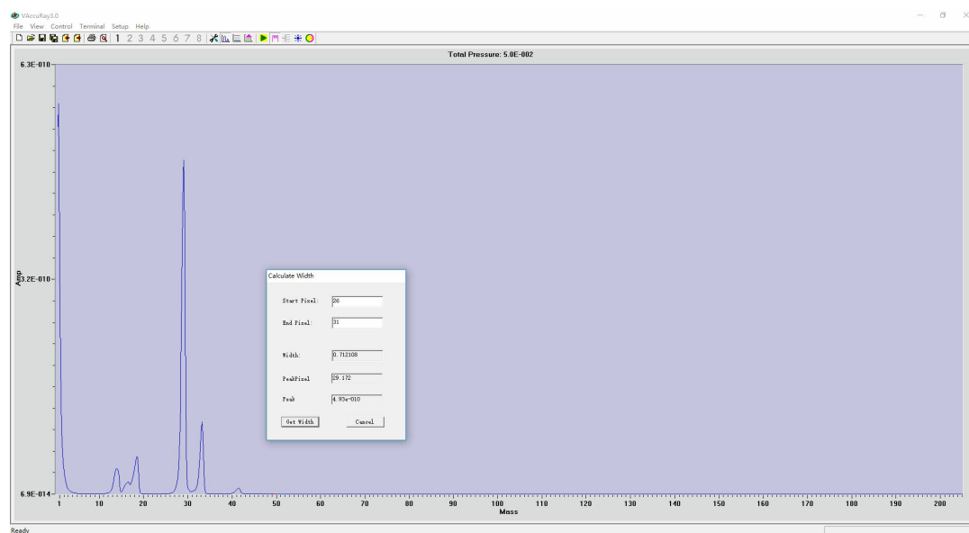
图 11: 真空度为 0.96 \times 10^{-2} Pa 改变分辨率为 60，电压为 40 下的扫描结果
