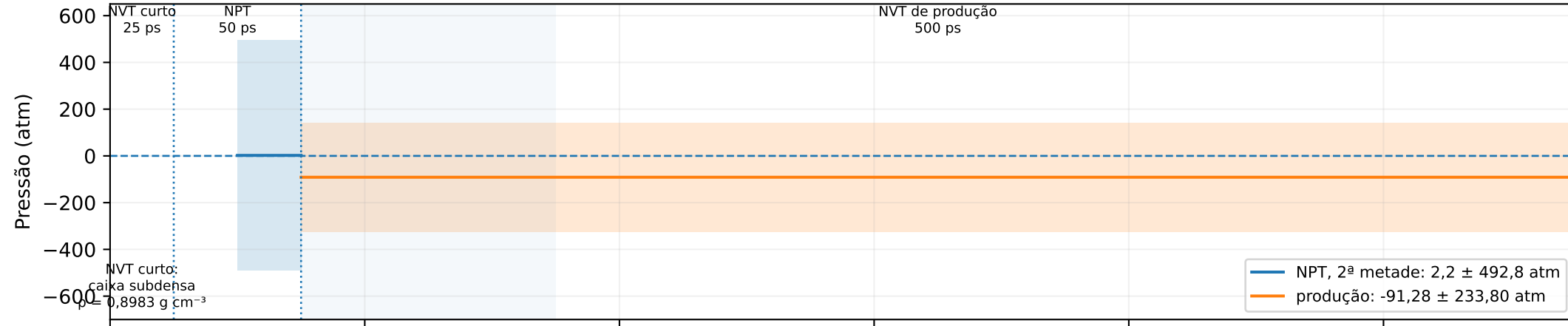
(c) Ajuste de densidade e volume fixo na produção
