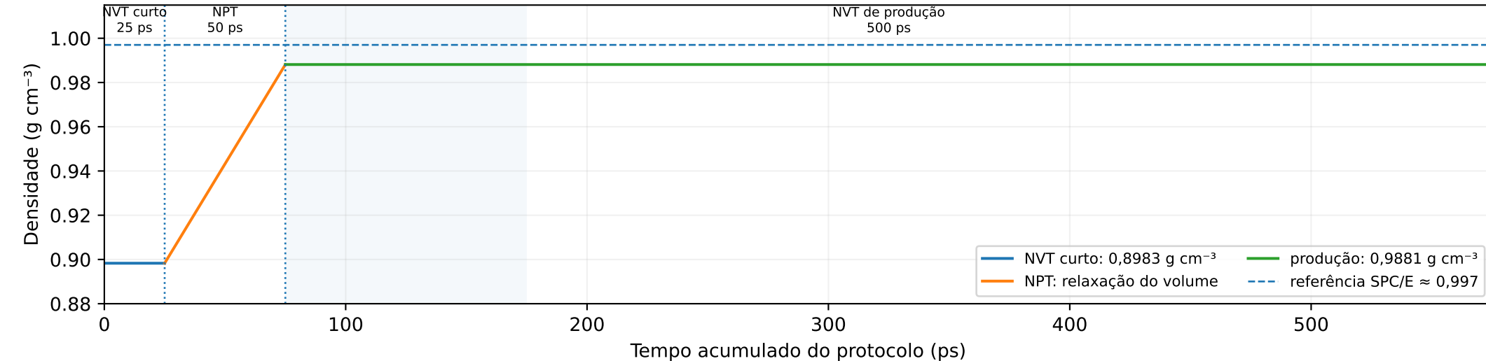
(c) Ajuste de densidade e volume fixo na produção
