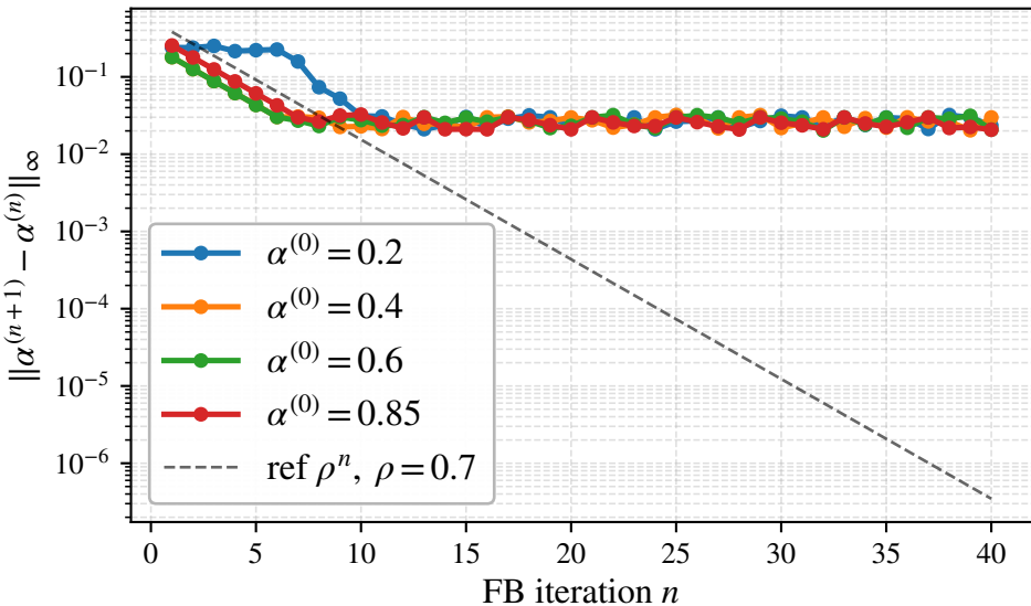
FB-PDE convergence (N=100, milan)
